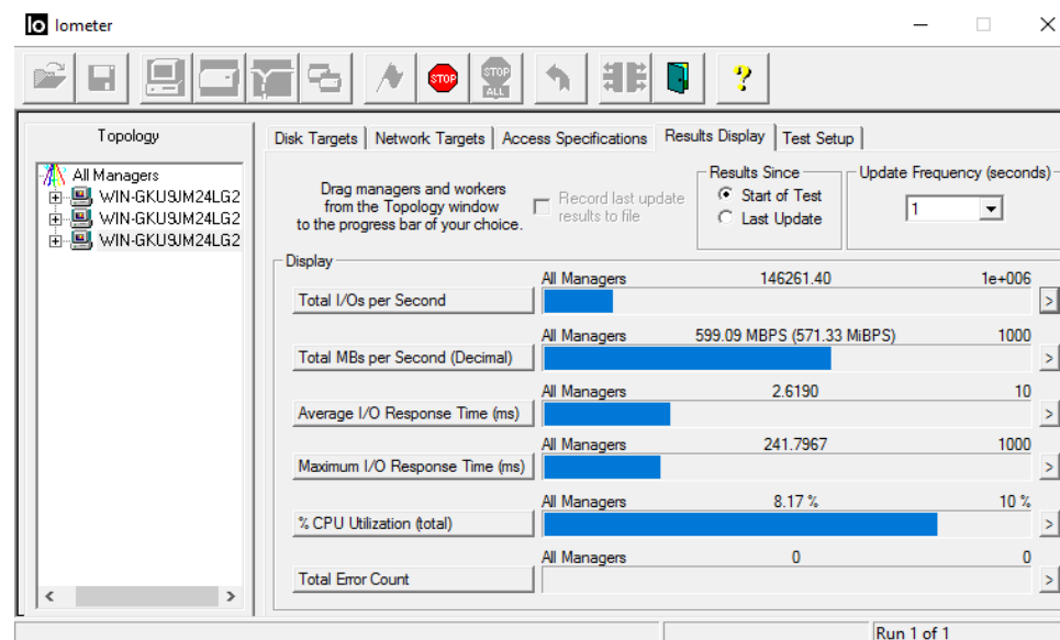
Последовательная запись блоков 4К, спустя 3 часа
