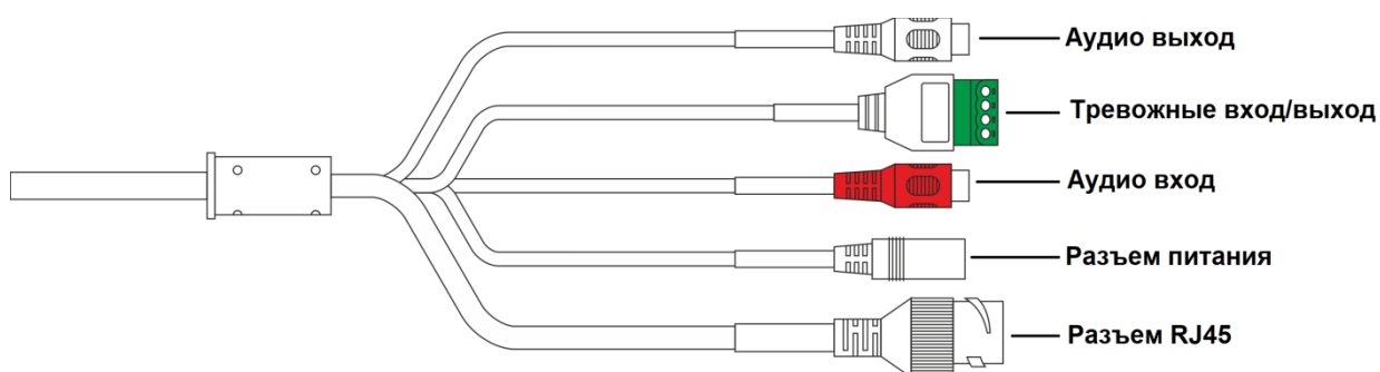
Рисунок 1. Коммутационный кабель
