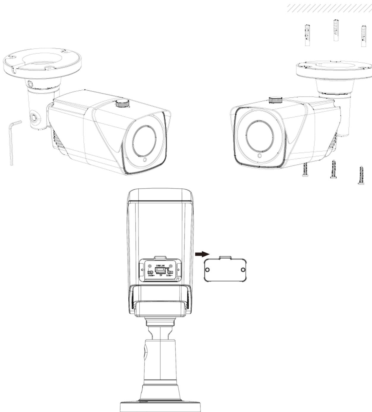
Рисунок 2. Монтаж камеры
