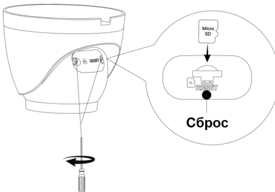
Рисунок 2. Монтаж камеры
