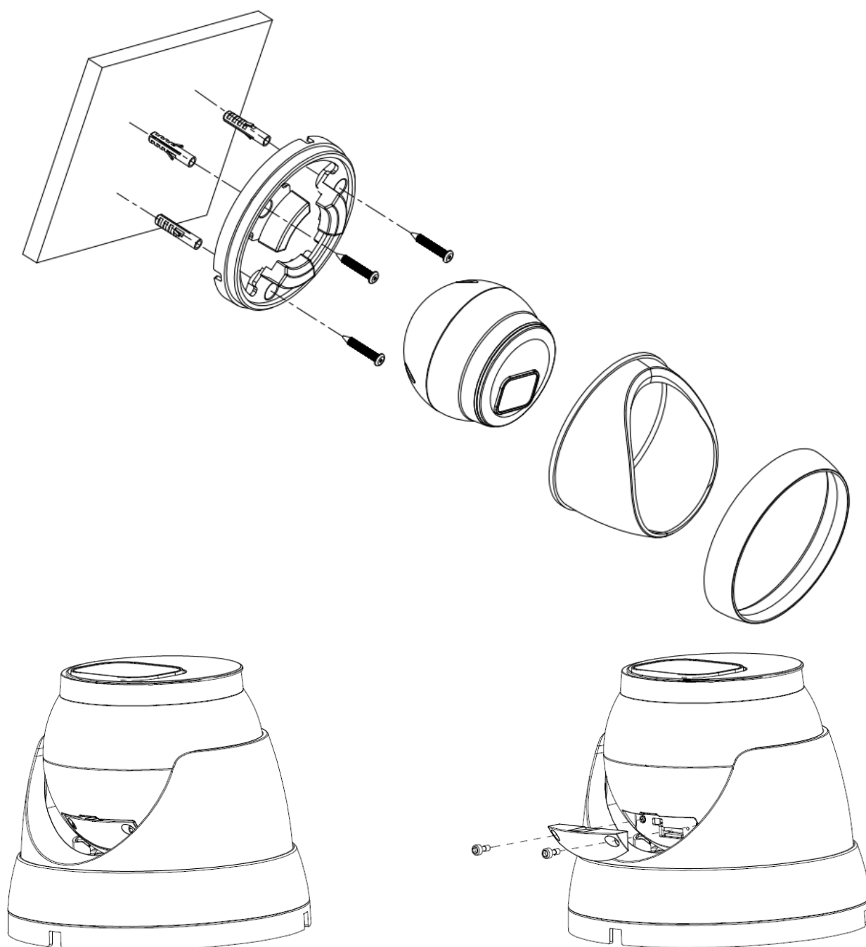
Рисунок 2. Монтаж камеры
