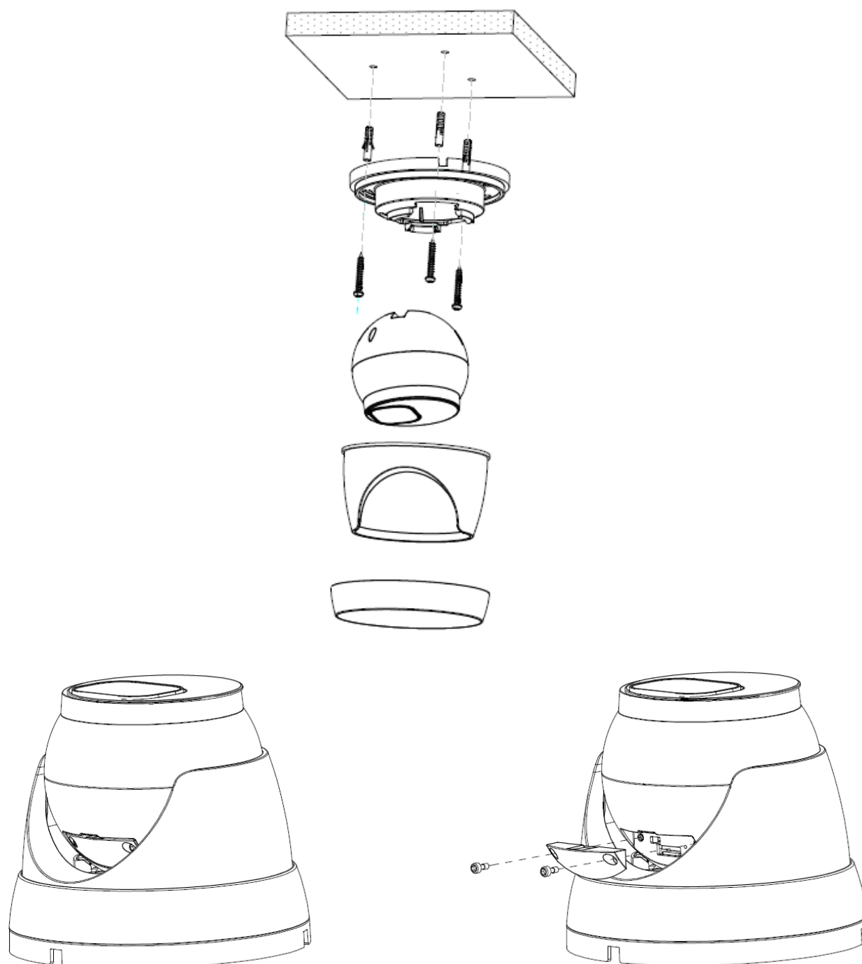
Рисунок 2. Монтаж камеры
