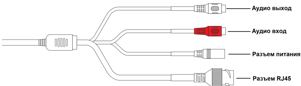
Рисунок 1. Коммутационный кабель
