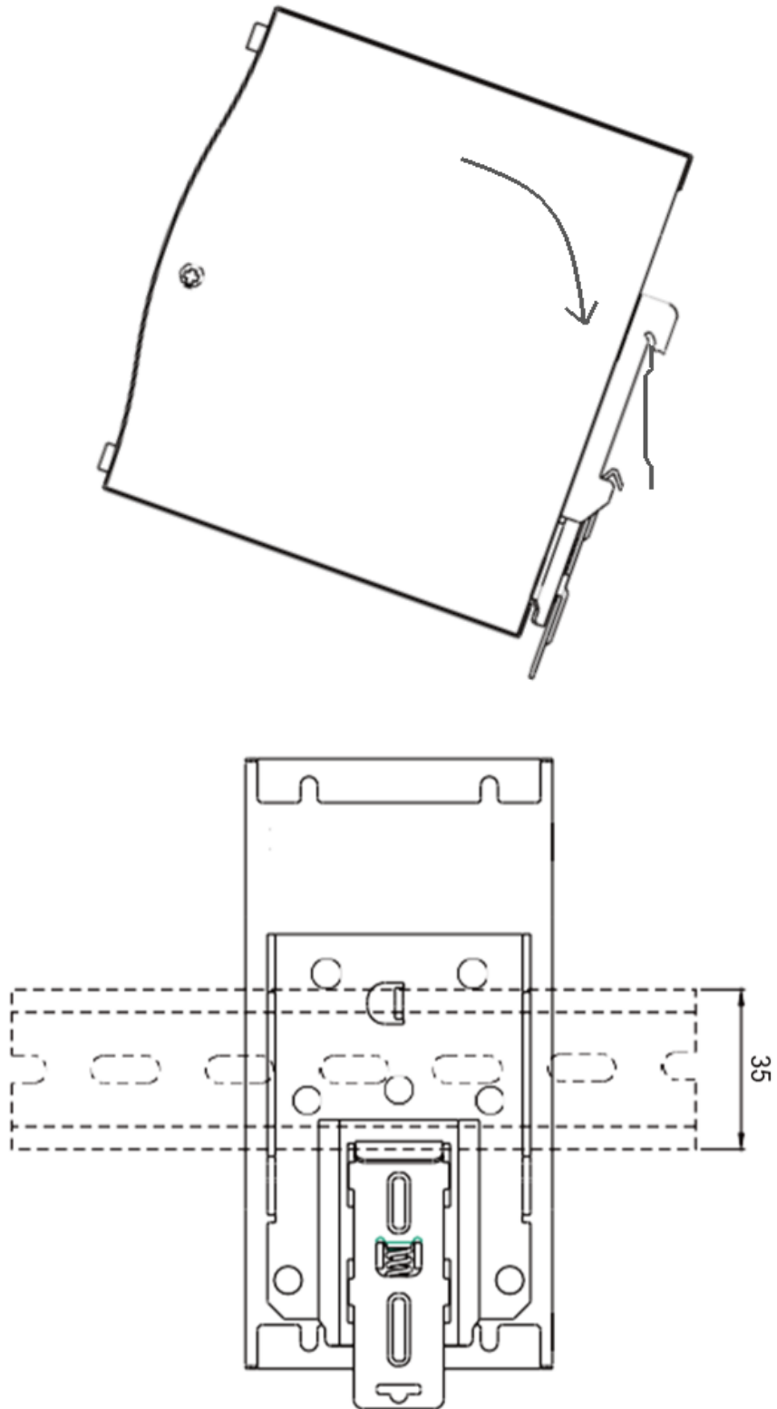
Рисунок 2. Монтаж на DIN-рейку
