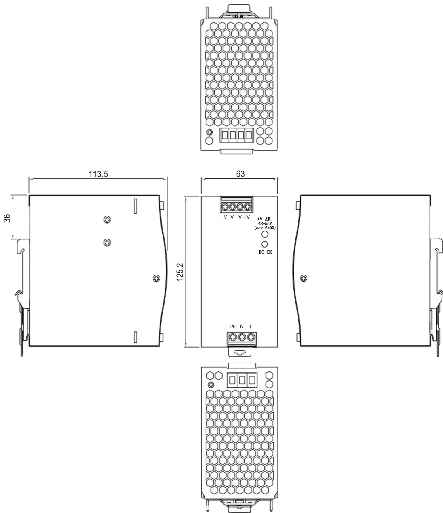
Рисунок 1. Вид сверху, слева, спереди, справа и снизу
