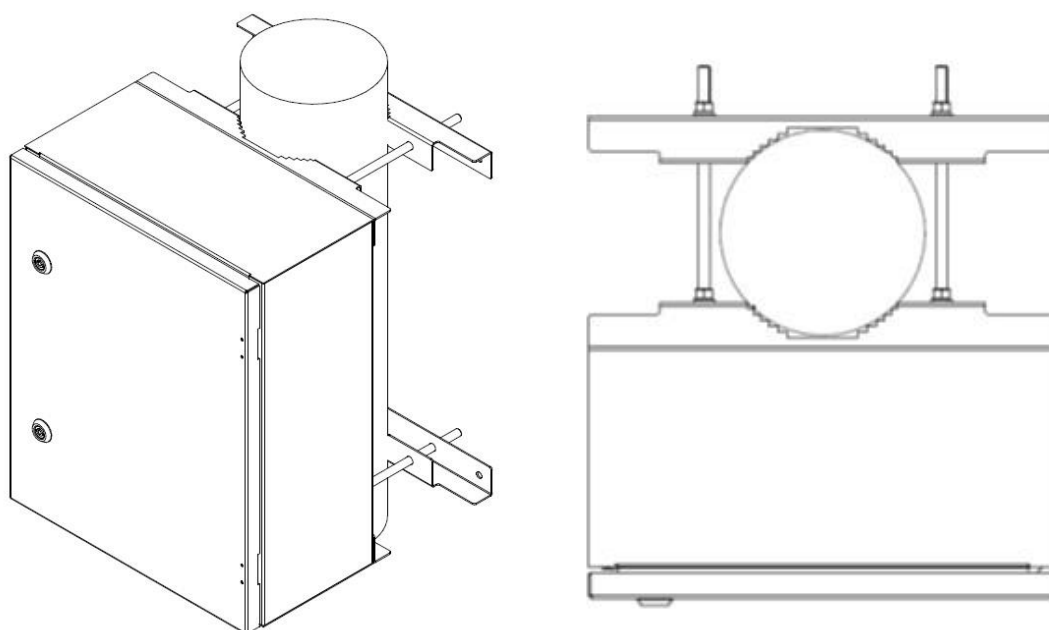
Рисунок 8-1. Установка шкафа на опору
