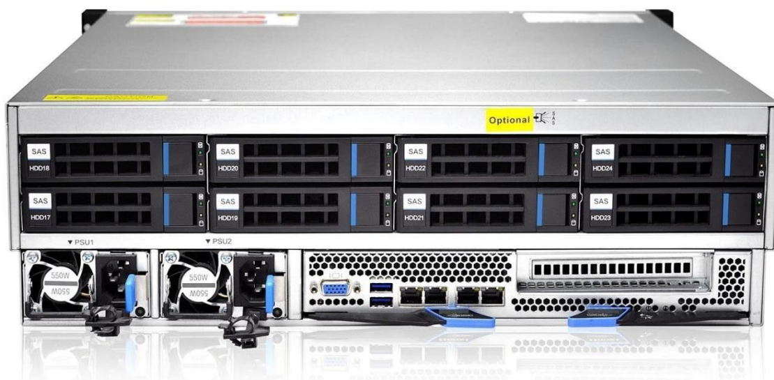
Рисунок 1. Серверная платформа QSRV-332404 (вид сзади)
