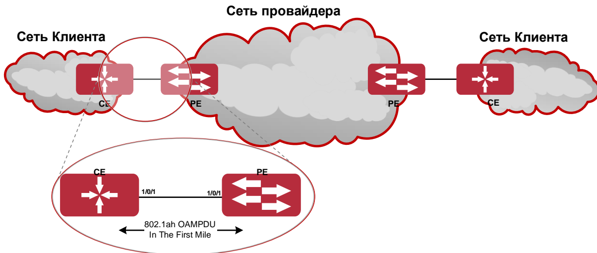
Рисунок 26. Типовая топология применения OAM
