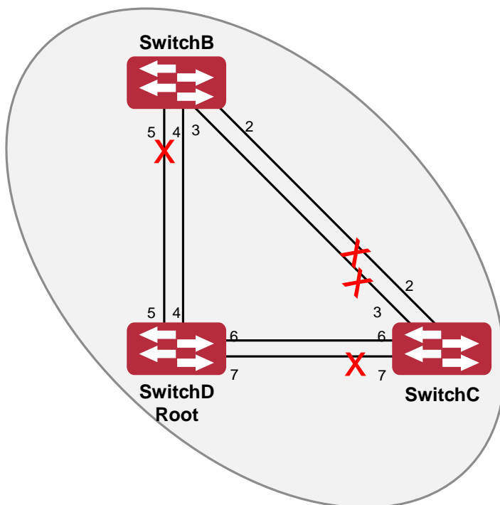
Рисунок 47. Топология экземпляра связующего дерева 4 после вычисления MSTP
