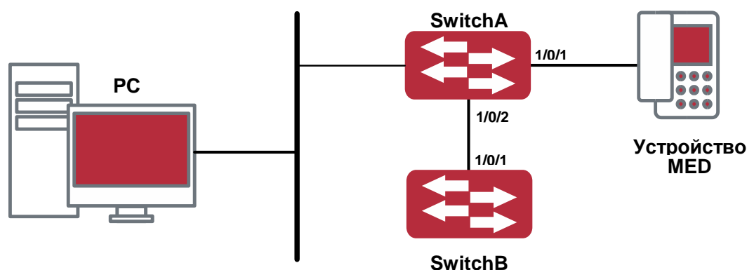
Рисунок 28. Топология базовой конфигурации LLDP-MED
