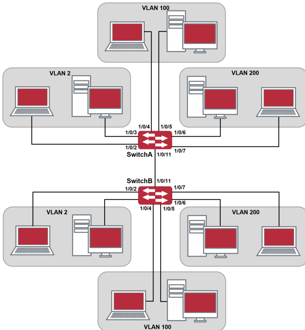
Рисунок 32. Типичная топология применения VLAN'а
