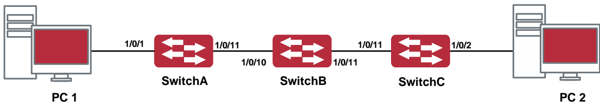
Рисунок 40. Типичная топология применения GVRP
