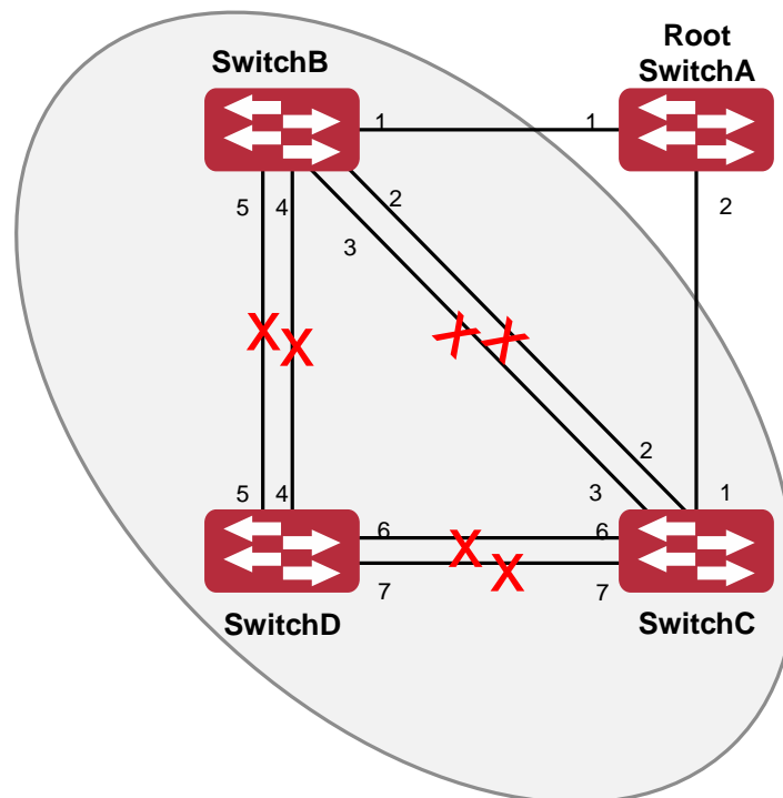
Рисунок 45. Топология экземпляра связующего дерева 0 после вычисления MSTP
