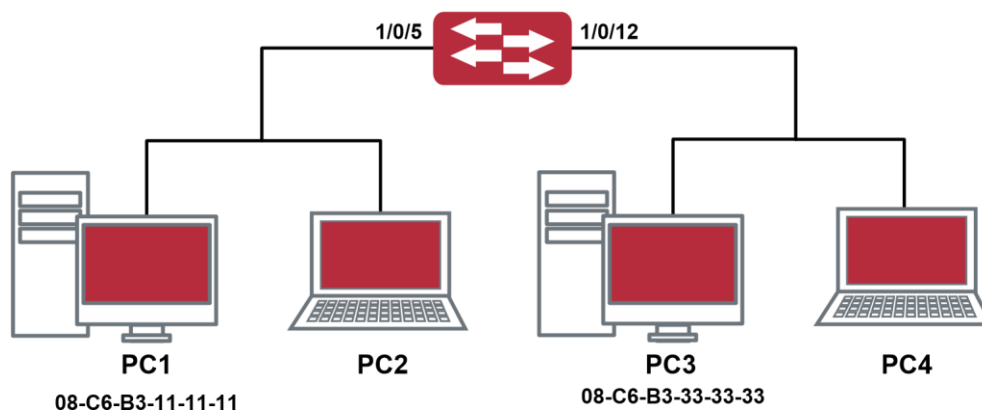
Рисунок 41. Динамическое построение таблицы MAC-адресов
