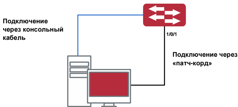
Рисунок 13. Типичная топология для обновления коммутатора в режиме BootROM
