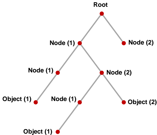
Рисунок 12. Пример дерева ASN.1
