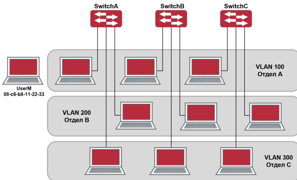
Рисунок 38. Типовая топология применения динамического VLAN'а
