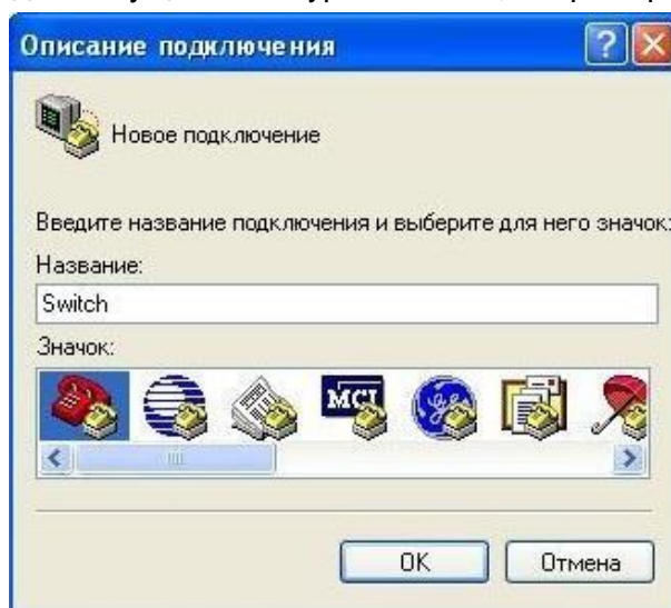
Рисунок 3. Запуск HyperTerminal.
