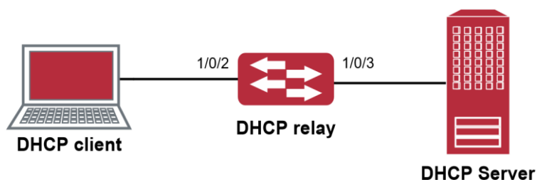
Рисунок 61. Конфигурация DHCP-ретранслятора
