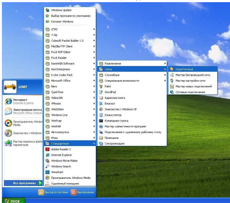
Рисунок 2. Запуск HyperTerminal.
