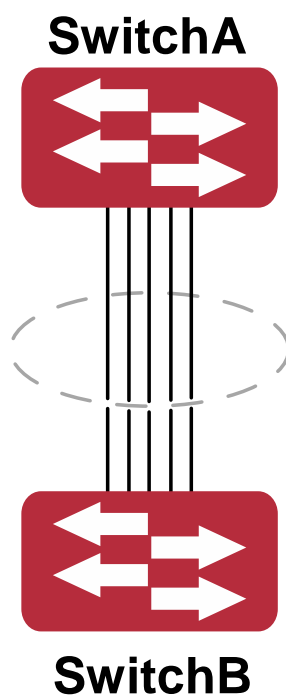
Рисунок 23. Конфигурация Port-Channel
