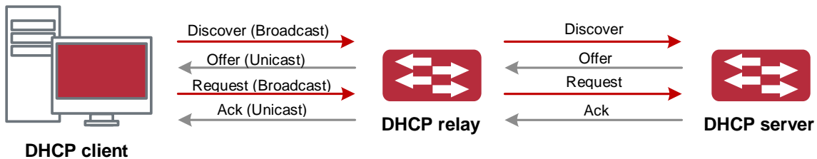
Рисунок 60. DHCP-ретранслятор
