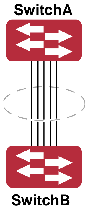
Рисунок 22. Агрегирование портов
