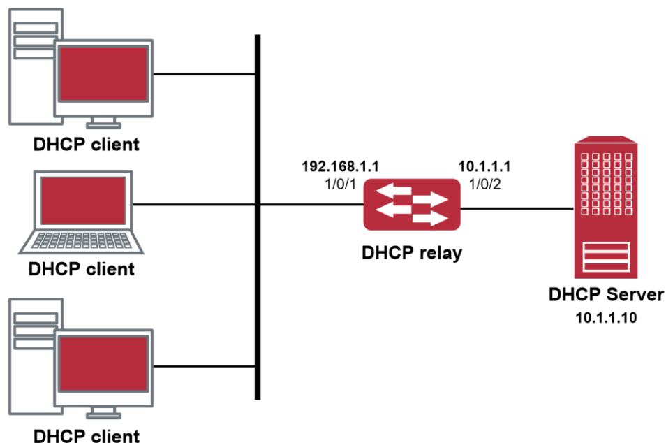
Рисунок 61. Конфигурация DHCP-ретранслятора
