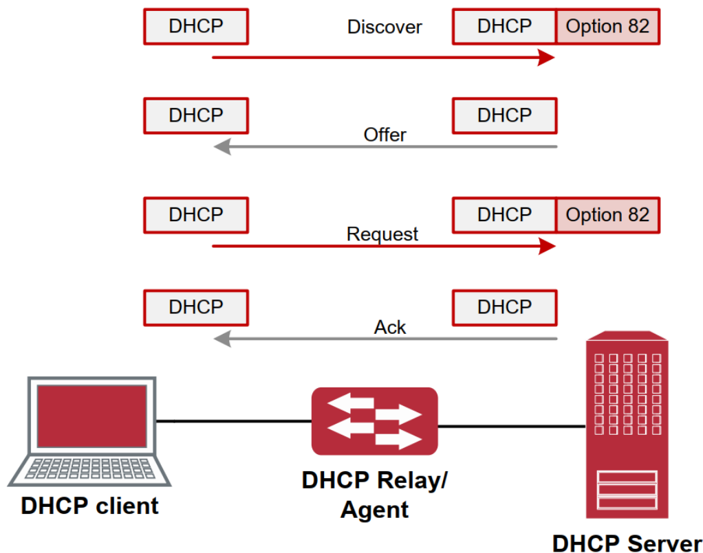
Рисунок 63. Диаграмма потоков опции 82 DHCP
