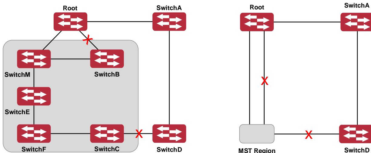
Рисунок 43. Пример CIST и региона MST
