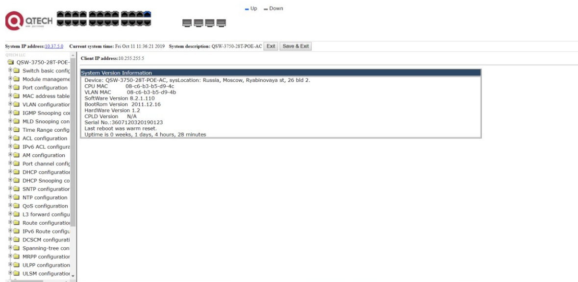
Рисунок 10. Управление Коммутатором
