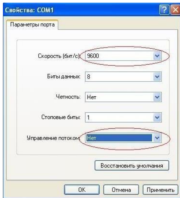
Рисунок 5. Запуск HyperTerminal.
