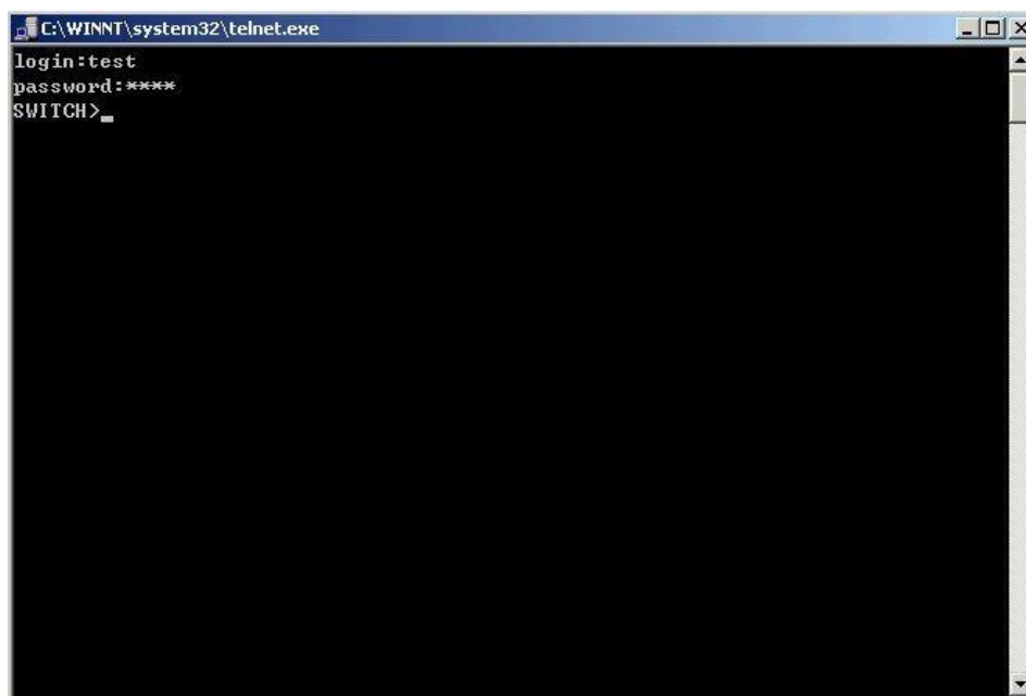
Рисунок 8. Настройка Telnet-интерфейса
