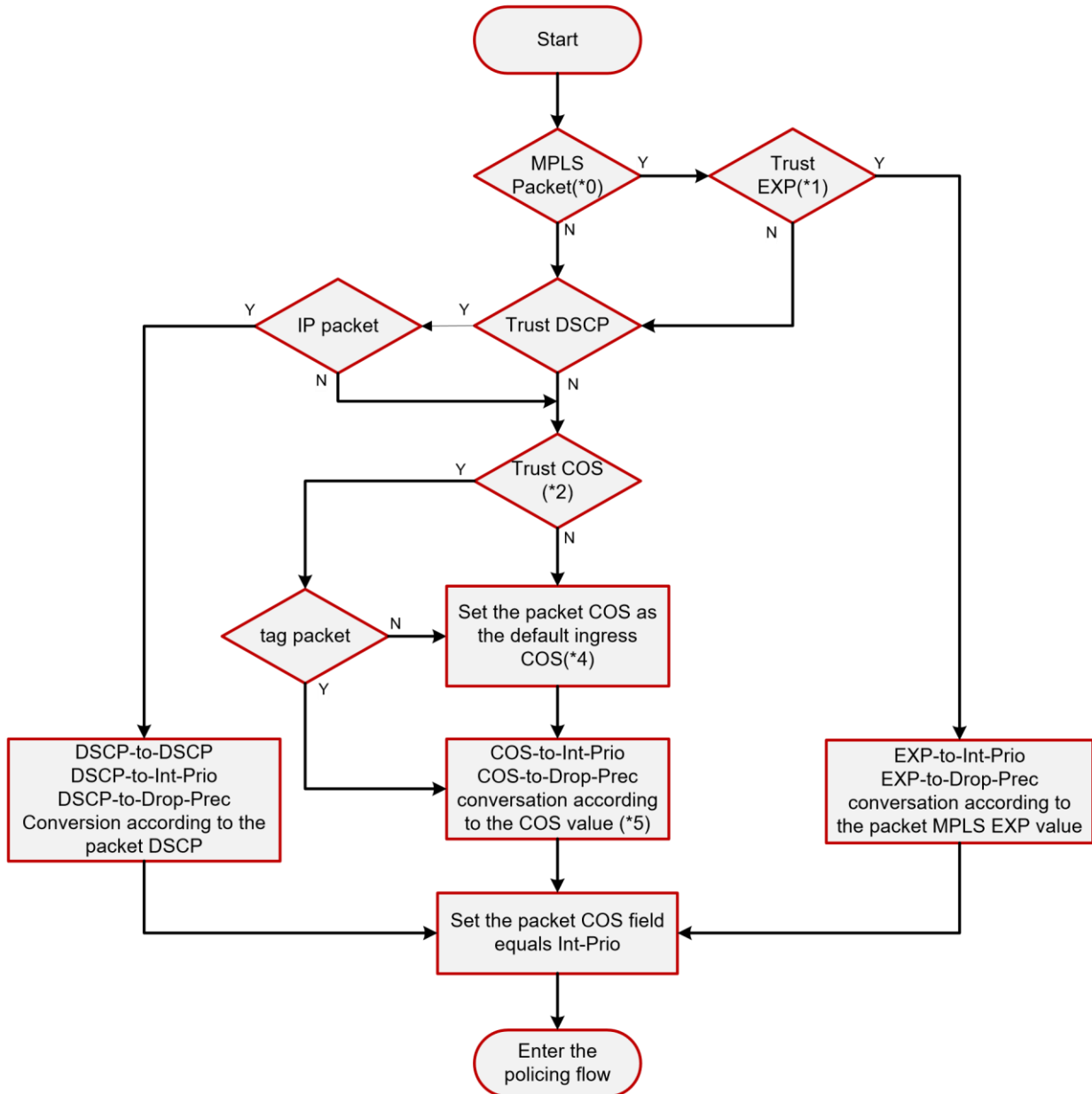
Рисунок 51. Процесс классификации
