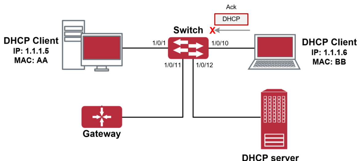
Рисунок 67. Типовой применение
