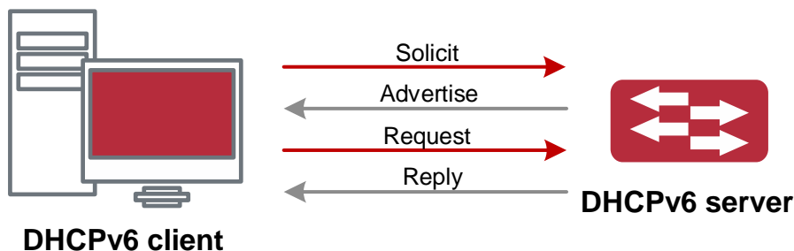
Рисунок 62. Согласование DHCPv6
