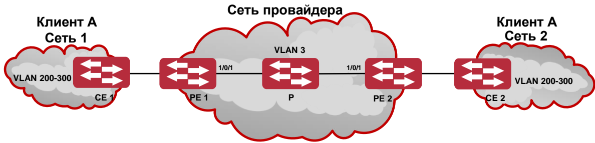
Рисунок 34. Межсетевое взаимодействие на основе Dot1q-туннеля
