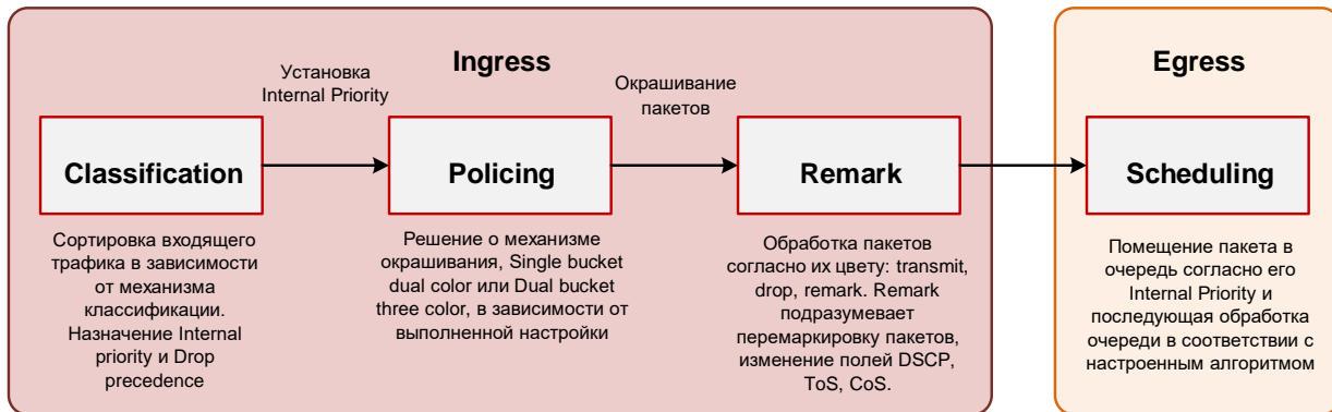
Рисунок 50. Базовая модель QoS
