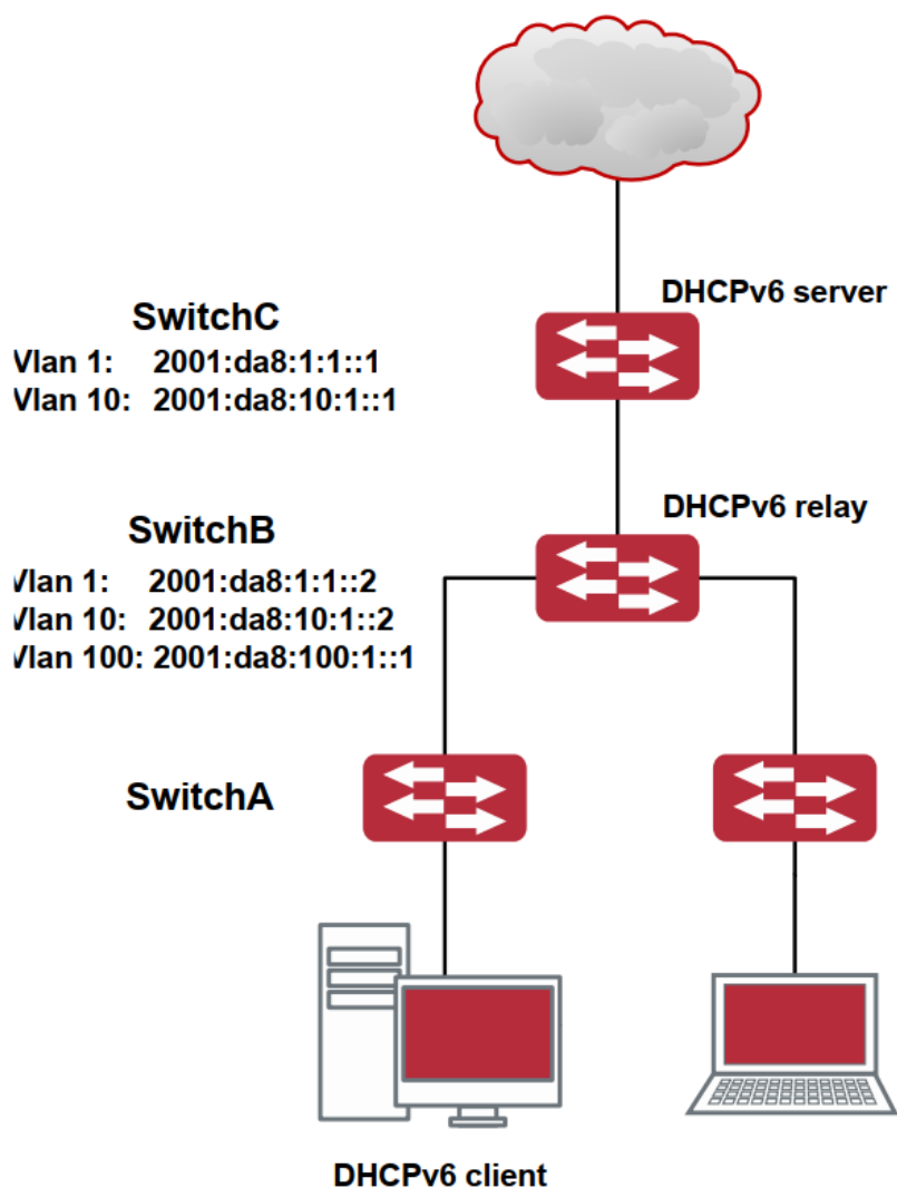
Рисунок 66. Схема применения опций в DHCPv6-ретрансляторе
