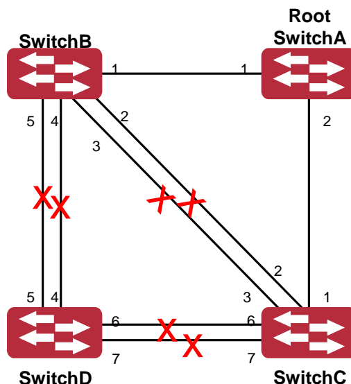
Рисунок 44. Типичный сценарий применения MSTP
