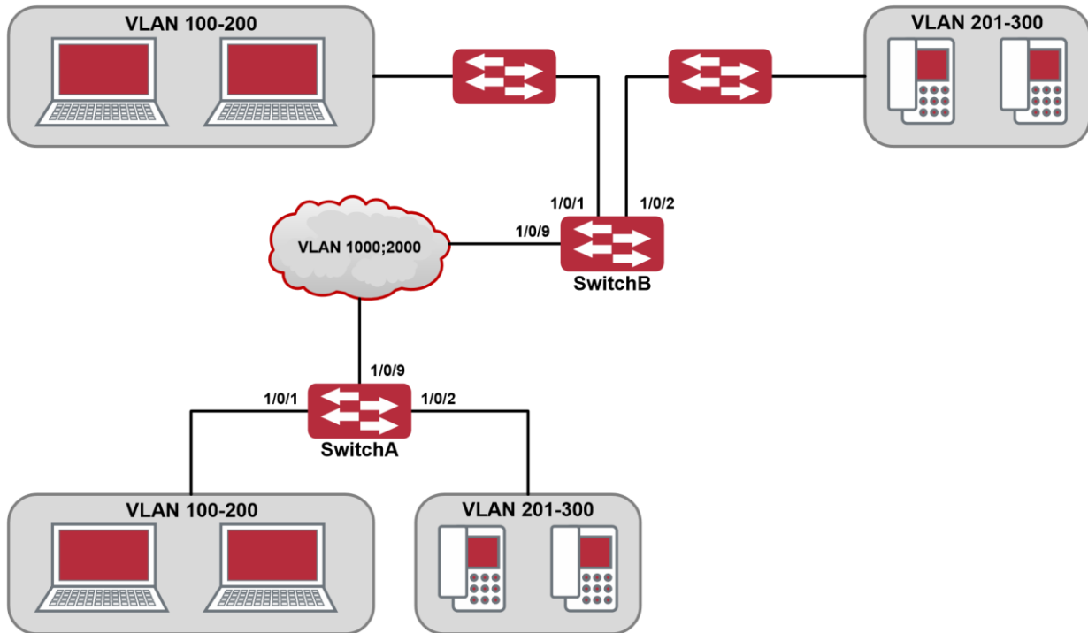
Рисунок 35. Применение Selective QinQ
