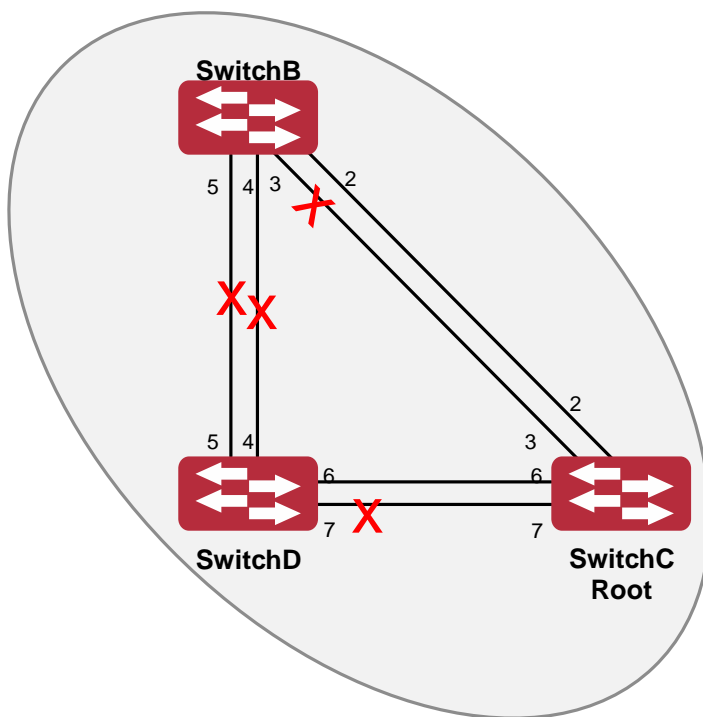
Рисунок 46. Топология экземпляра связующего дерева 3 после вычисления MSTP
