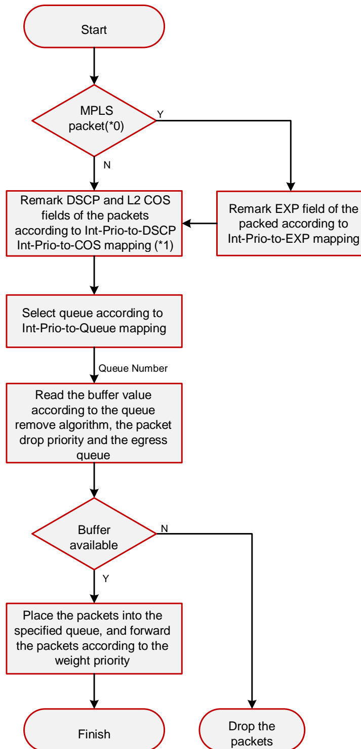
Рисунок 53. Процессы планировки и управления очередями
