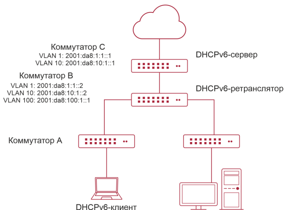
Рисунок 30-2. Схема применения опций в DHCPv6-ретрансляторе
