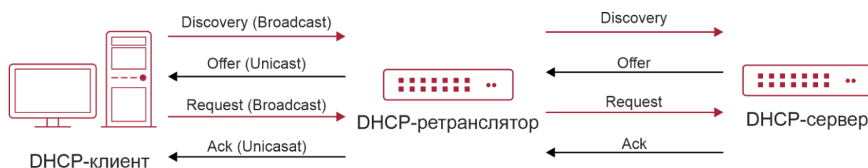
Рисунок 26-2. DHCP-ретранслятор
