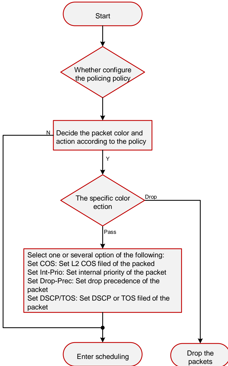
Рисунок 18-5. Процессы Регулирования и пометки
