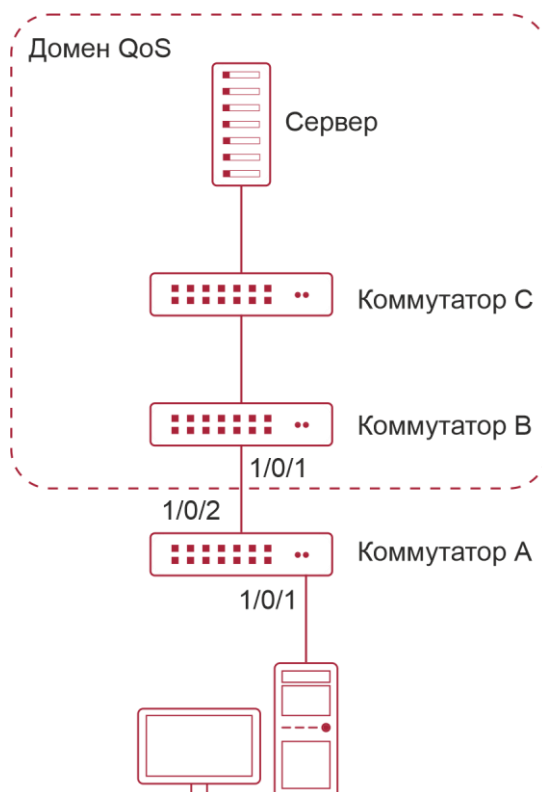
Рисунок 18-7. Типовая топология QoS
