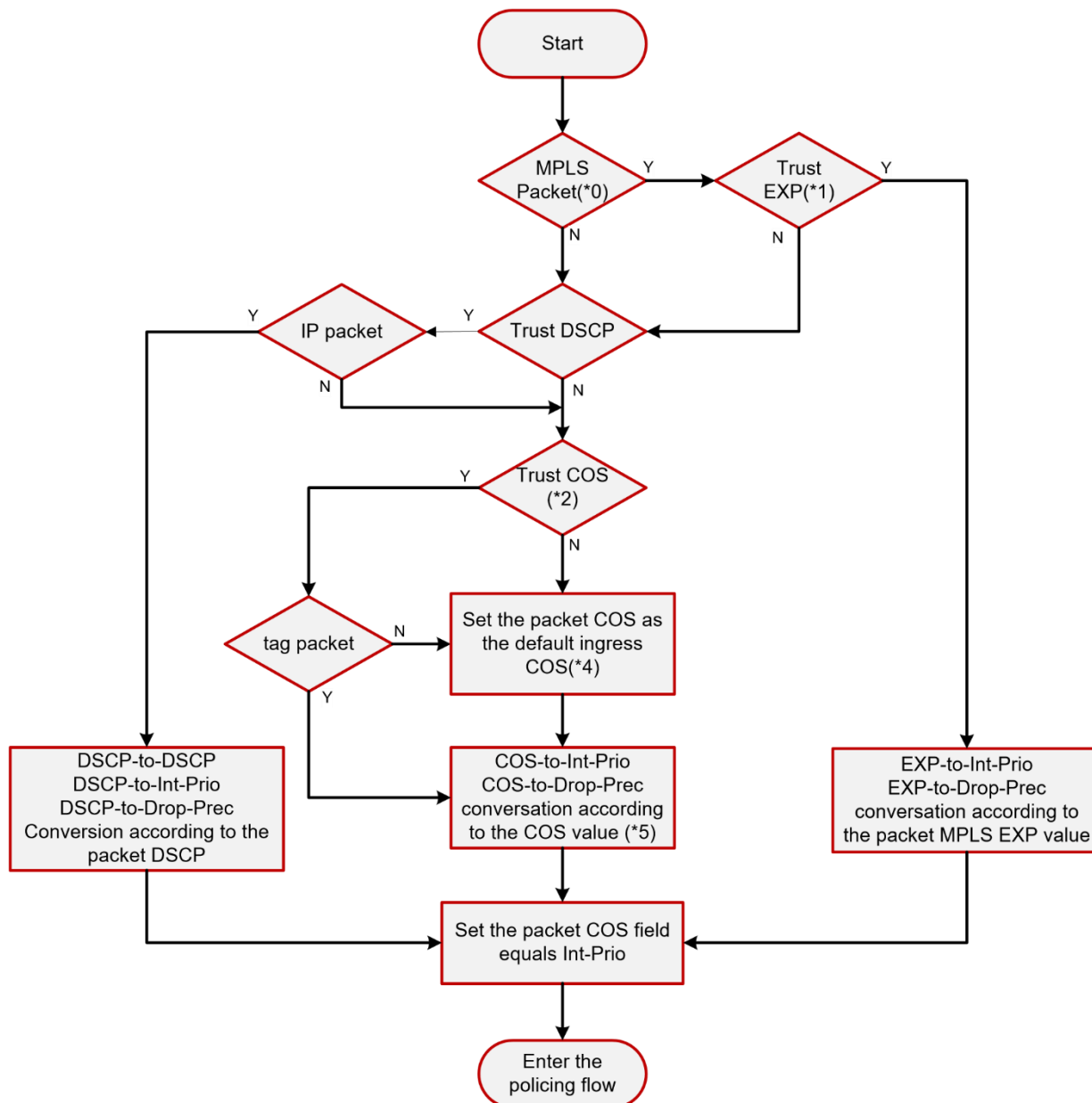
Рисунок 18-4. Процесс классификации
