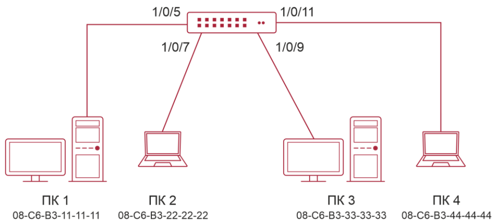
Рисунок 16-2. Типичный пример конфигурации таблицы MAC-адресов
