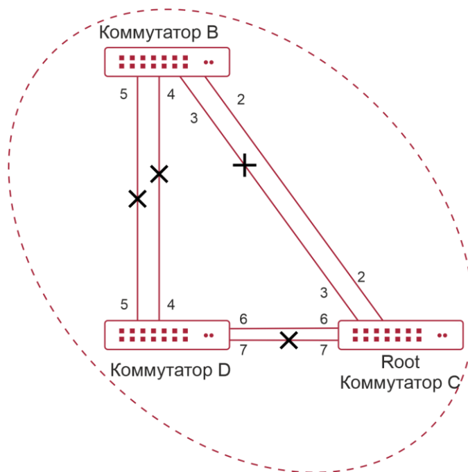
Рисунок 17-4. Топология экземпляра связующего дерева 3 после вычисления MSTP
