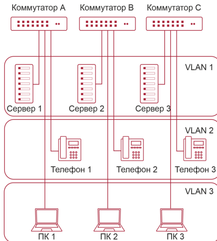
Рисунок 15-1. Логическое определение сети VLAN
