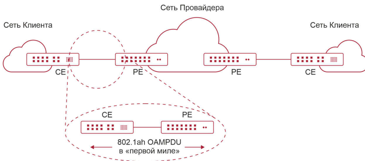
Рисунок 10-2. Типовое применение OAM-топологии
