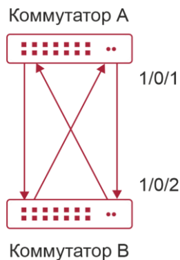
Рисунок 6-1. Перекрестное подключение двунаправленного оптического соединения
