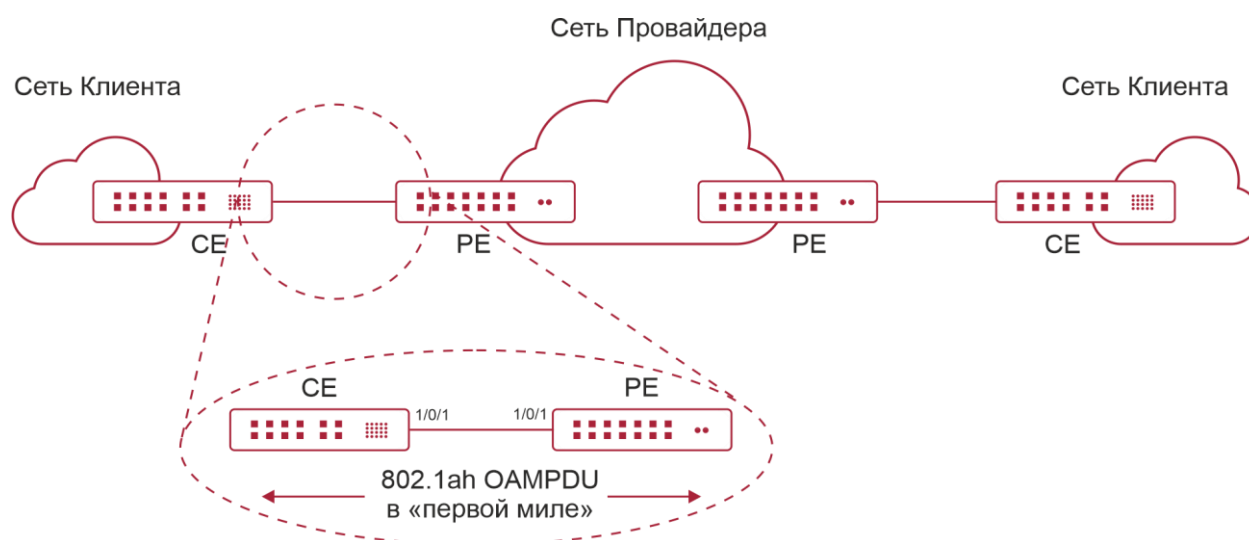
Рисунок 10-3. Типовая топология применения OAM
