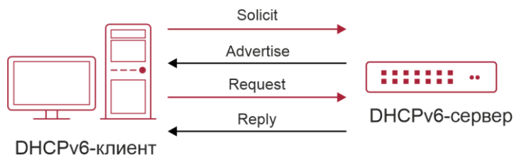
Рисунок 27-1. Согласование DHCPv6
