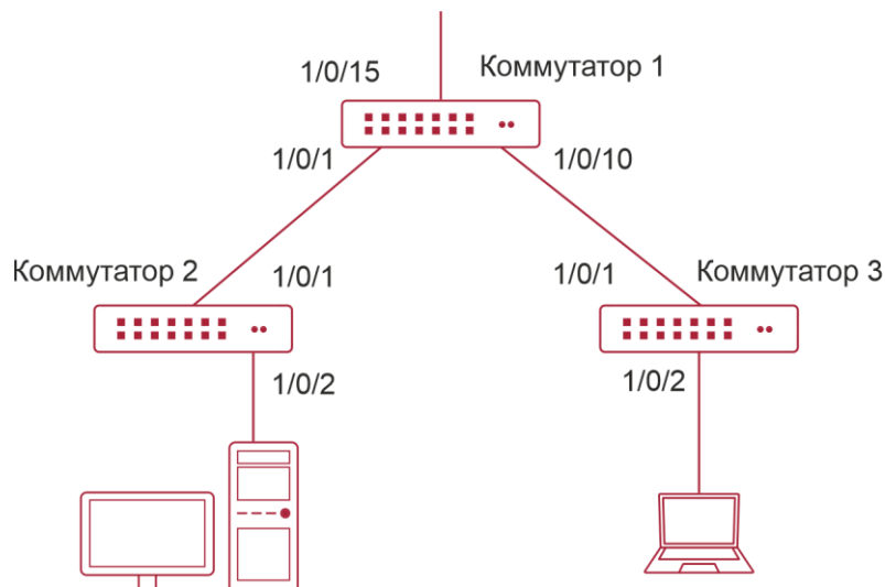
Рисунок 4-1. Типовые примеры функции изоляции портов
