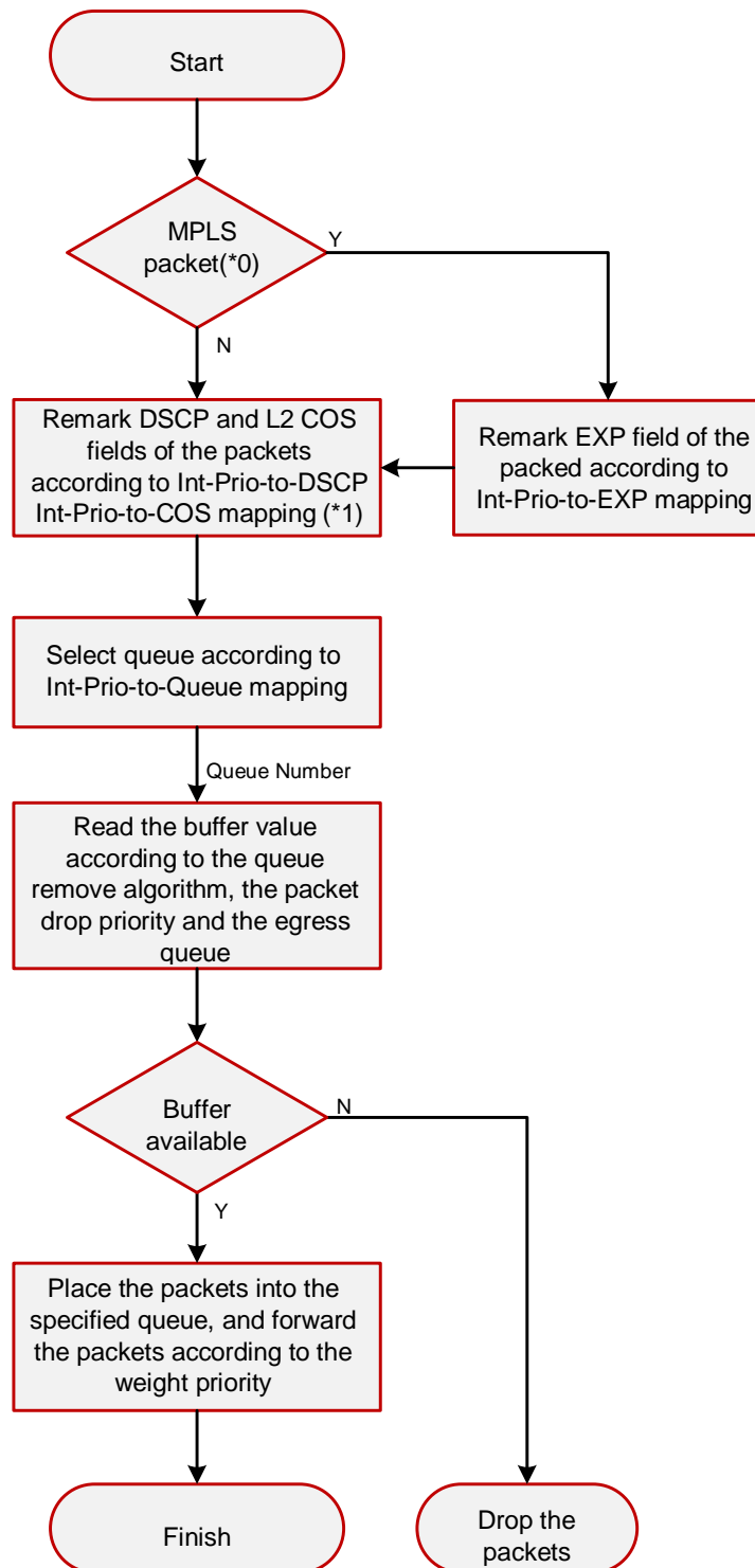
Рисунок 18-6. Процессы планировки и управления очередями
