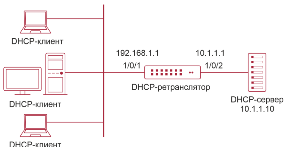
Рисунок 26-3. Конфигурация DHCP-ретранслятора
