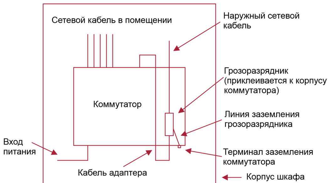
Рисунок 7-2. Схематическая диаграмма грозозащитника на Ethernet-порте
