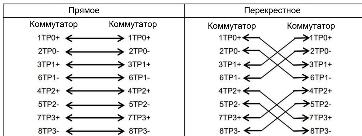
Рисунок 6-1. Четыре витых пары для порта 1000 BASE-T
