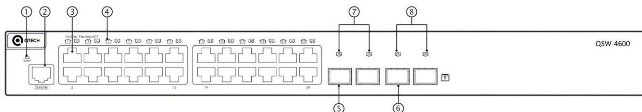
Рисунок 1-1. Передняя панель QSW-4600-28TX
