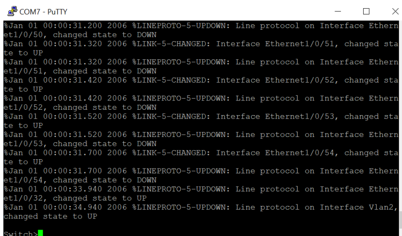
Рисунок 4-6. Коммутатор загрузился
