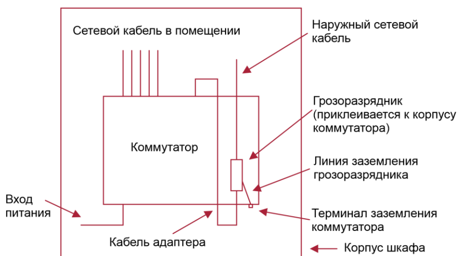
Рисунок 8-2. Схематическая диаграмма грозоразрядника на Ethernet-порту
