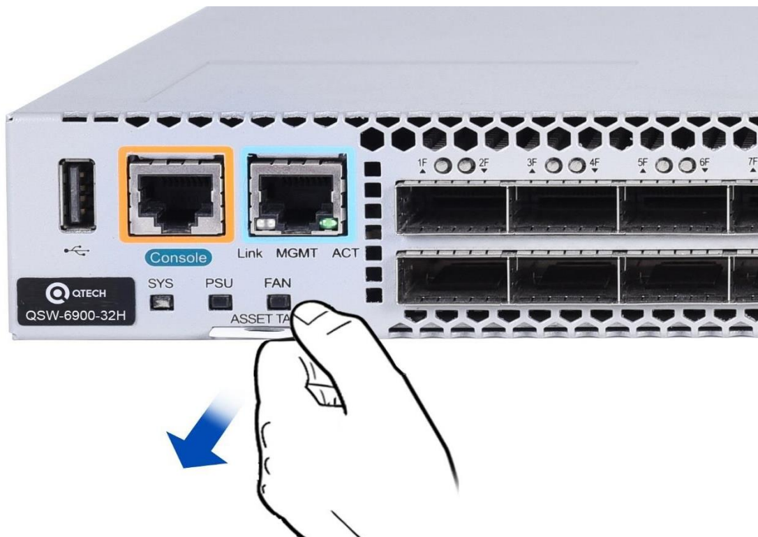
Рисунок 1-4. Маркировка коммутатора QSW-6900-32H
