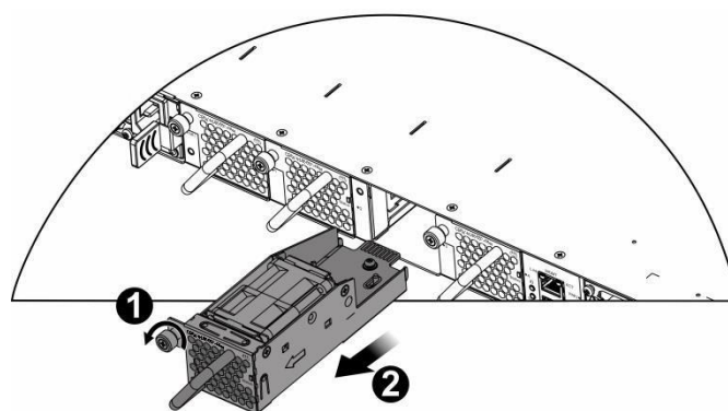
Рисунок 3-4. Извлечение модуля вентилятора
