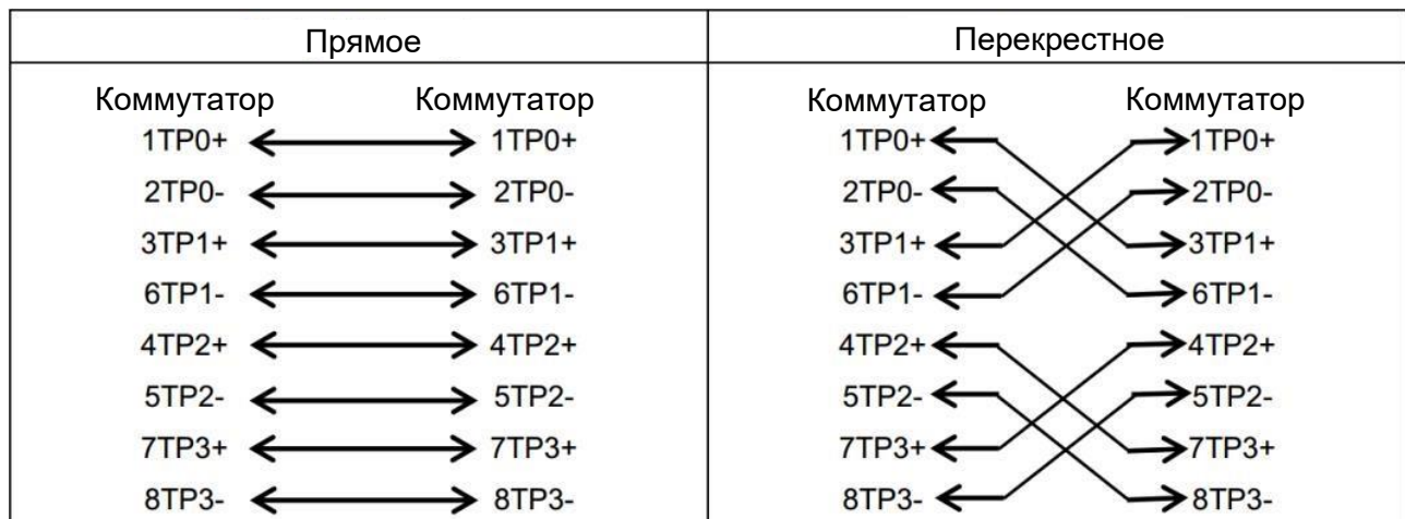
Рисунок 7-1. Четыре витых пары для порта 1000 BASE-T
