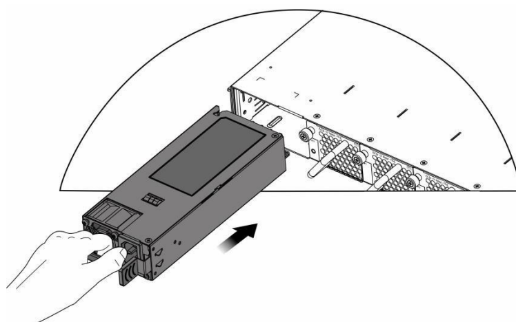
Рисунок 3-5. Установка модуля питания
