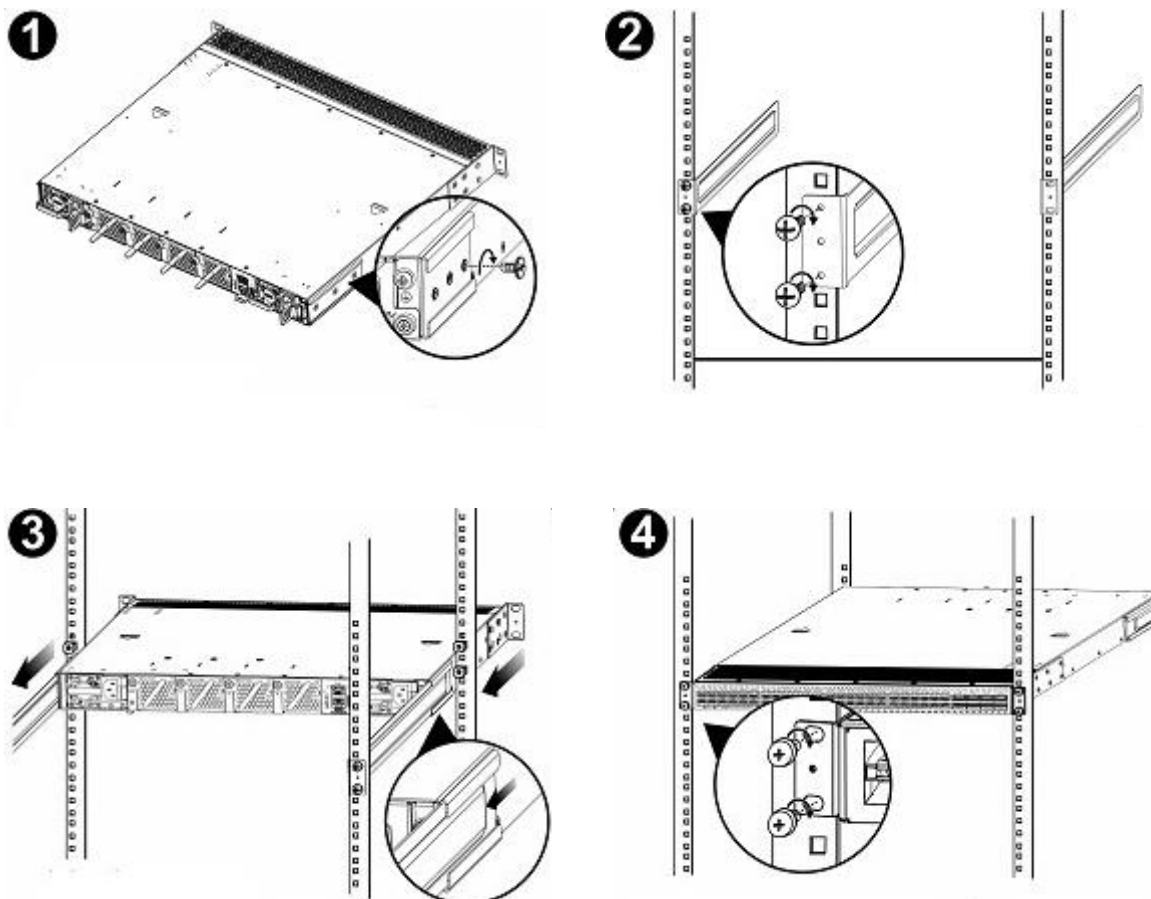
Рисунок 3-2. Установка коммутатора в стойку
