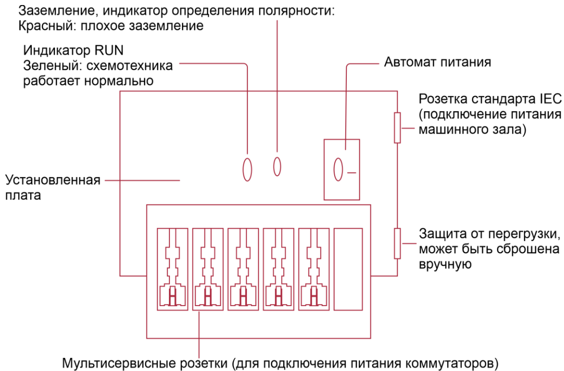
Рисунок 8-1. Схематическая диаграмма автомата питания
