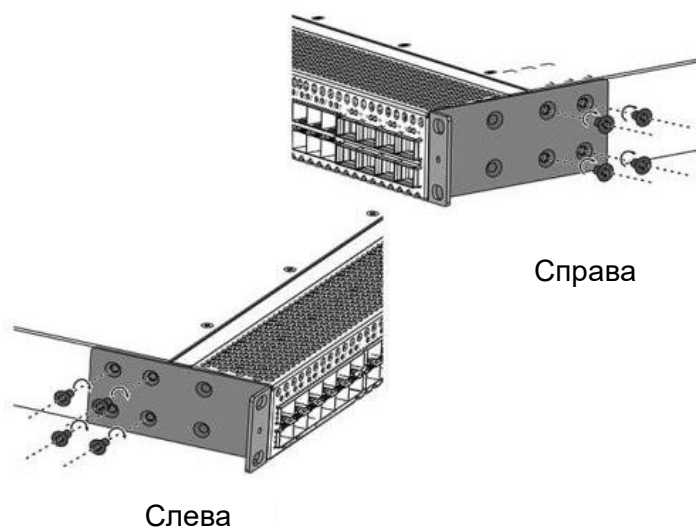
Рисунок 3-1. Установка монтажных кронштейнов
