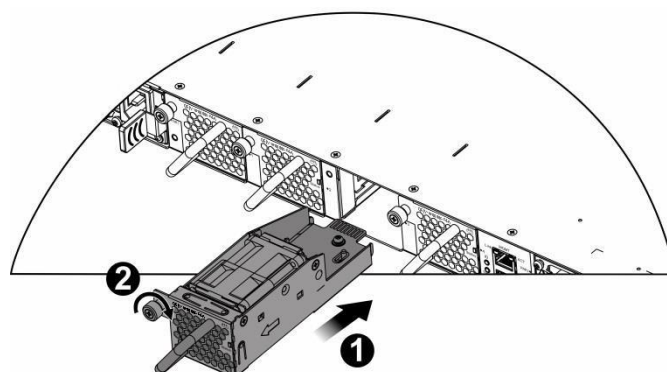
Рисунок 3-3. Установка модуля вентилятора панели модуля вентилятора, чтобы избежать неправильной установки.
