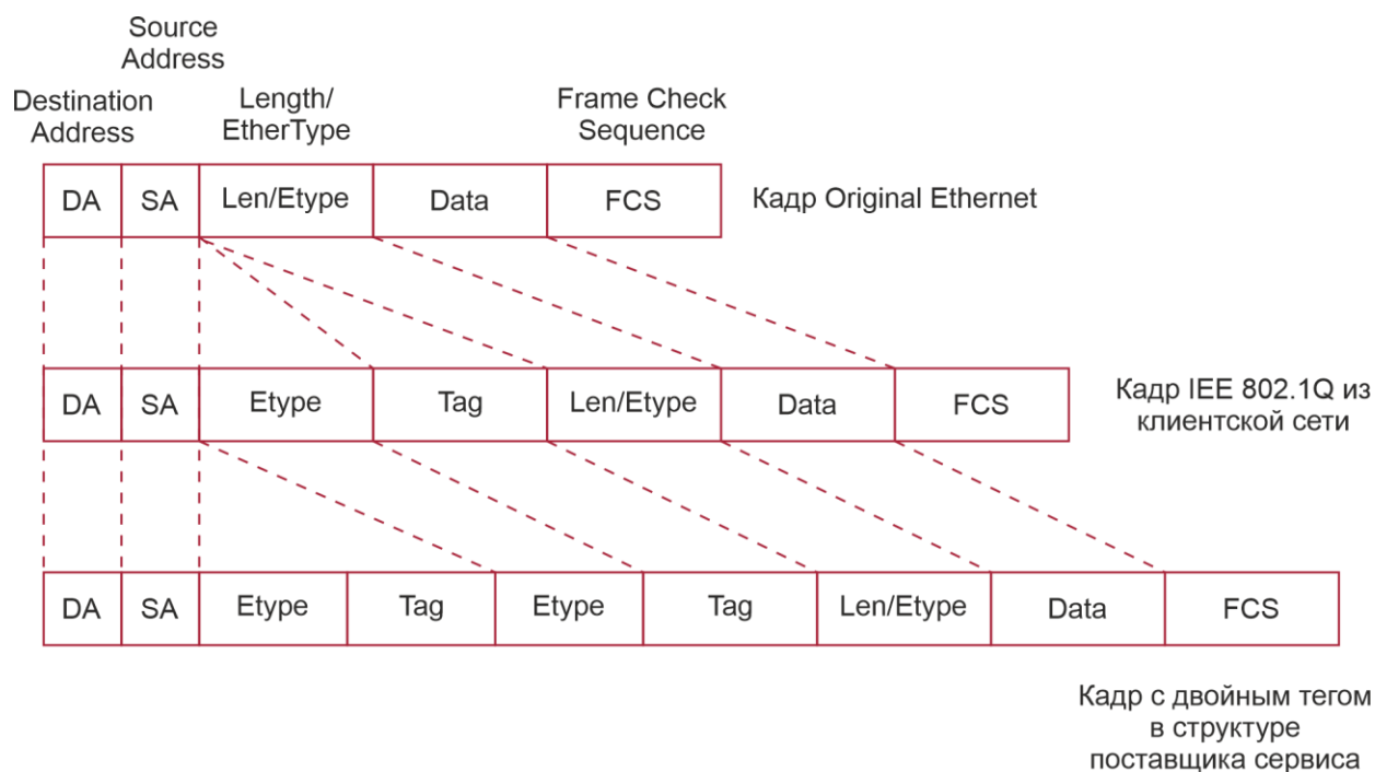
Рисунок 13-1. Инкапсуляция внешнего тега
