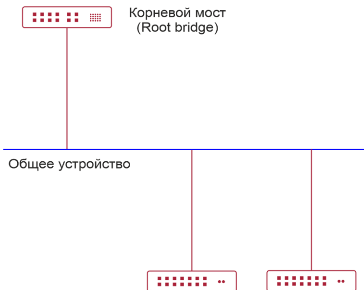
Рисунок 10-8. Пример соединения не «точка-точка»
