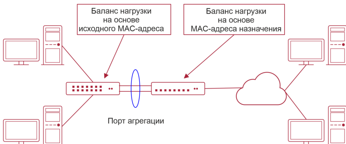
Рисунок 4-1. Агрегация каналов AP и балансировка нагрузки
