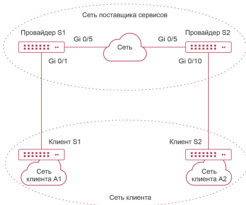
Рисунок 11-2. Топология туннельных приложений GVRP PDU
