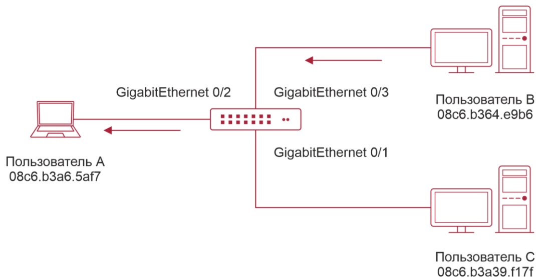
Рисунок 3-2. Шаг 2. Изучение MAC-адреса
