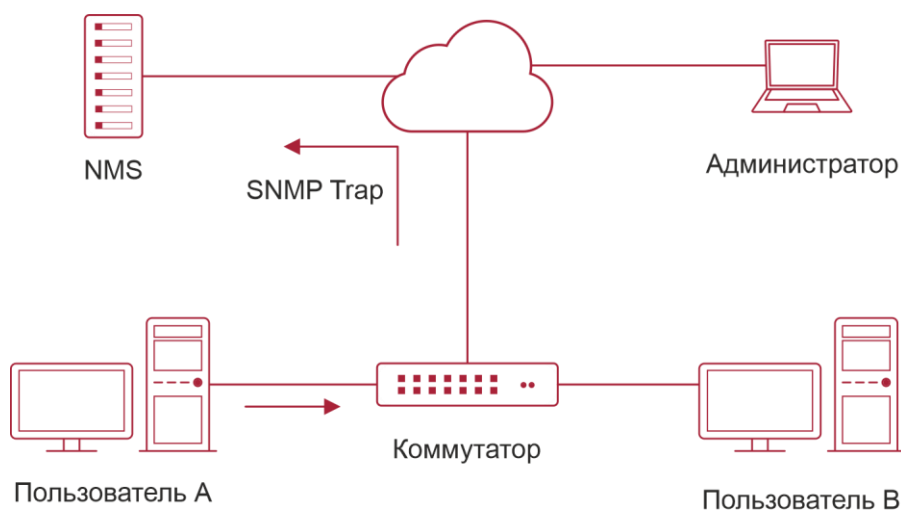
Рисунок 3-3. Уведомление об изменении MAC-адреса
