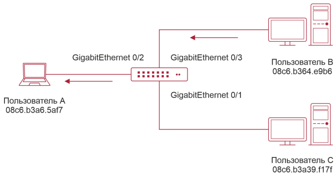
Рисунок 3-1. Шаг 1. Изучение MAC-адреса
