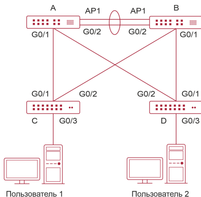
Рисунок 10-1. Dual-Core топология MSTP+VRRP
