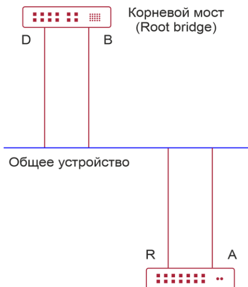
Рисунок 10-7. Пример соединения не «точка-точка»
