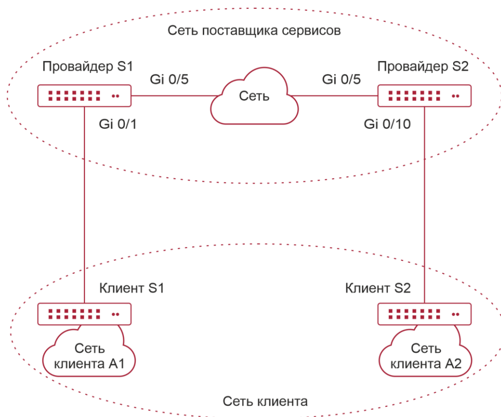
Рисунок 10-2. Топология туннеля BPDUTunnel
