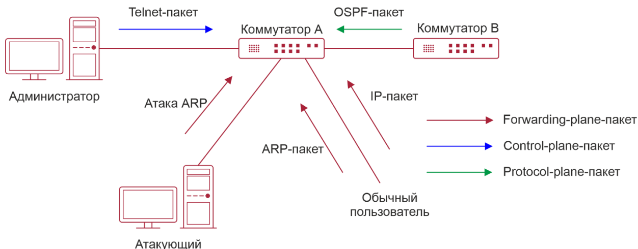
Рисунок 9-1. Сетевая топология коммутаторов и атак
