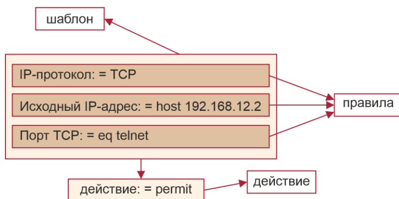
Рисунок 1-2. Анализ ACE: permit tcp host 192.168.12.2 any eq telnet
