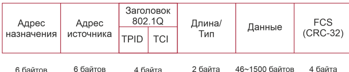
Рисунок 2-3. Структура пакета уровня 2
