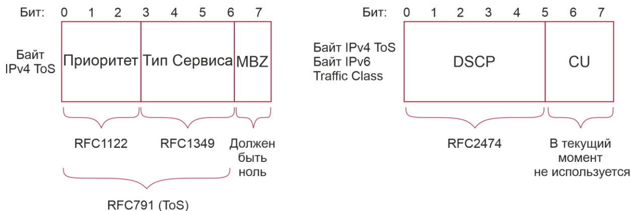
Рисунок 2-4. Расположение приоритетов IP PRE и DSCP в пакетах IPv4/IPv6
