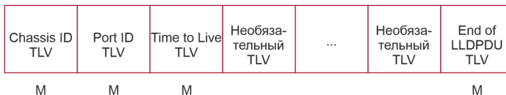
Рисунок 10-3. Формат LLDPDU
