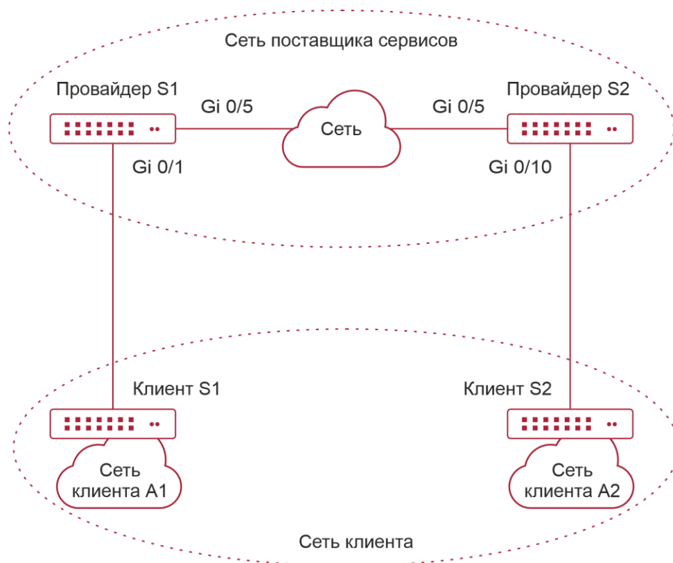
Рисунок 9-2. Топология туннельных приложений GVRP PDU
