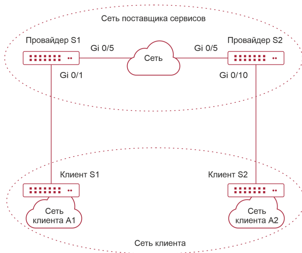
Рисунок 8-2. Топология туннеля BPDU
