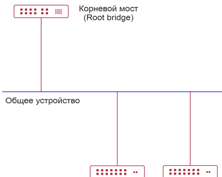
Рисунок 8-8. Пример соединения не «точка-точка»
