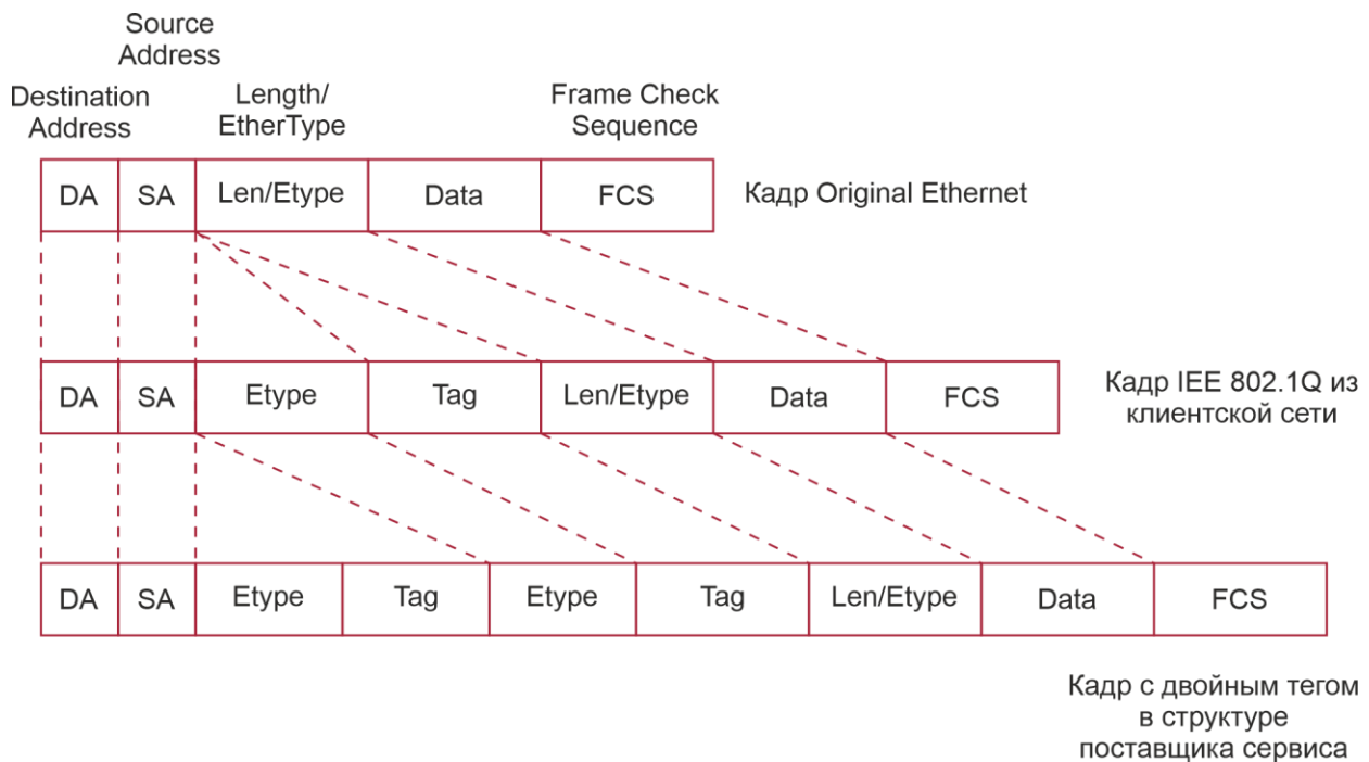
Рисунок 11-1. Инкапсуляция внешнего тега
