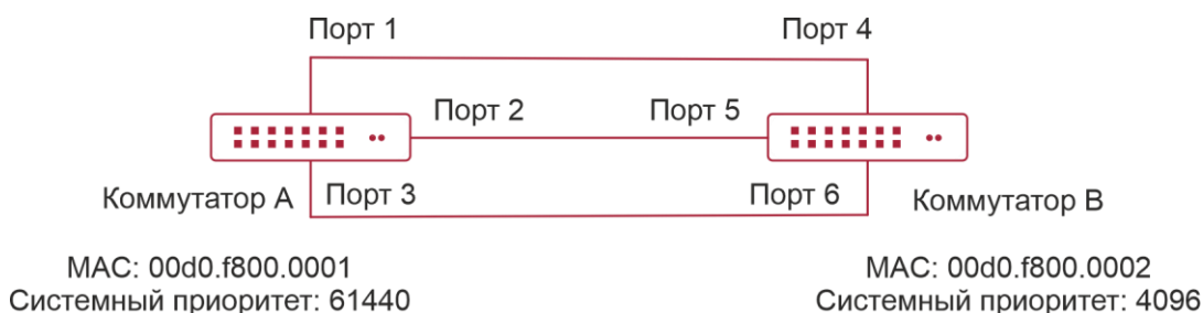
Рисунок 4-2. LACP-согласование
