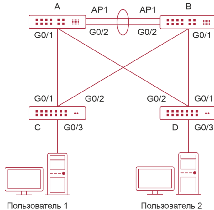
Рисунок 8-1. Dual-Core топология MSTP+VRRP
