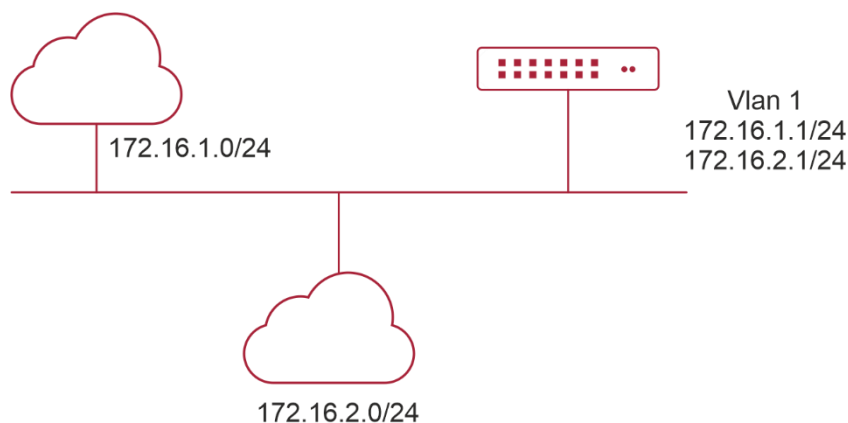
Рисунок 1-1. Настройка IP-адресов
