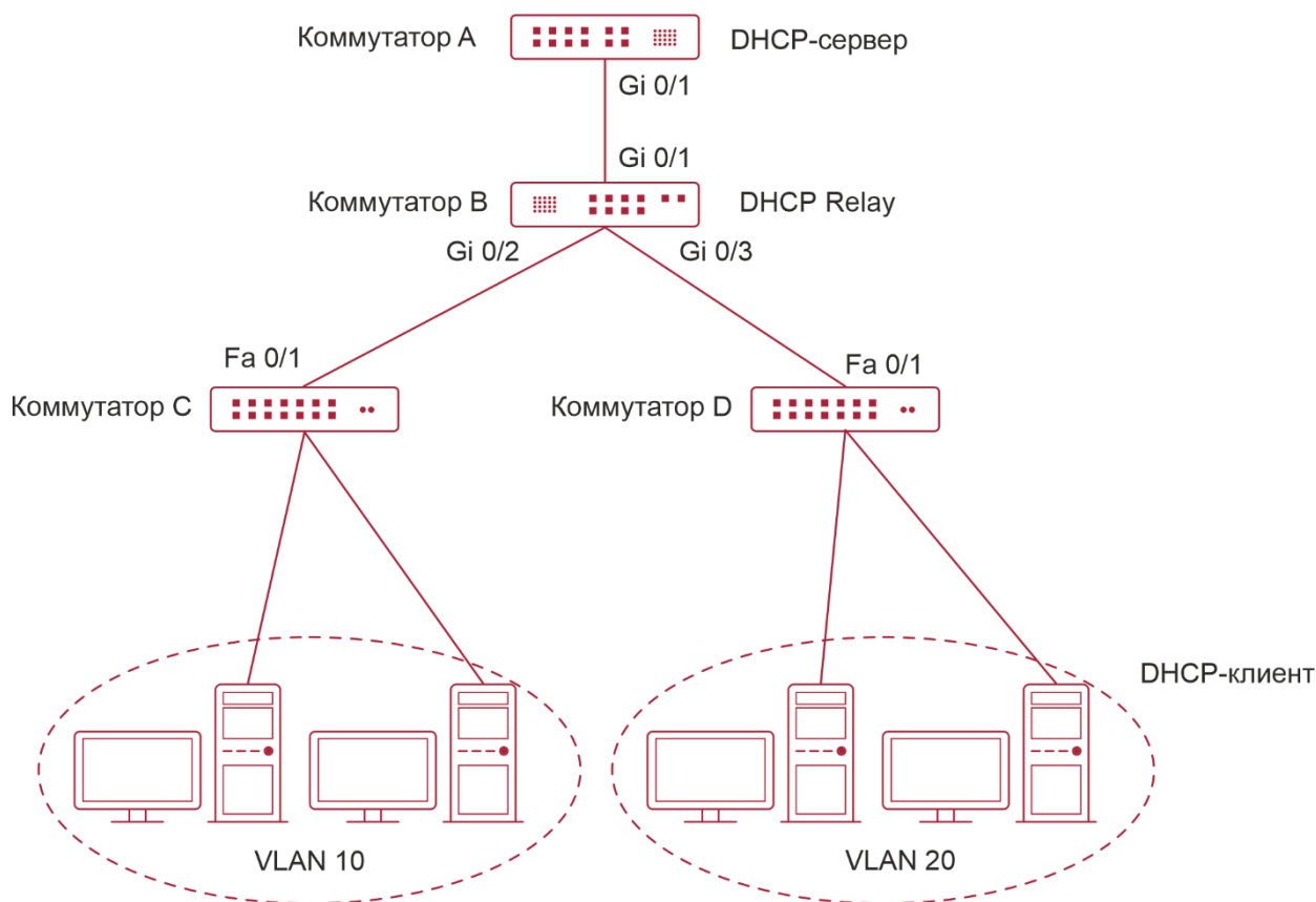
Рисунок 4-4. DHCP Relay
