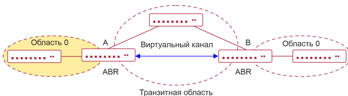
Рисунок 4-4. Прерывистая магистральная область в физической сети
