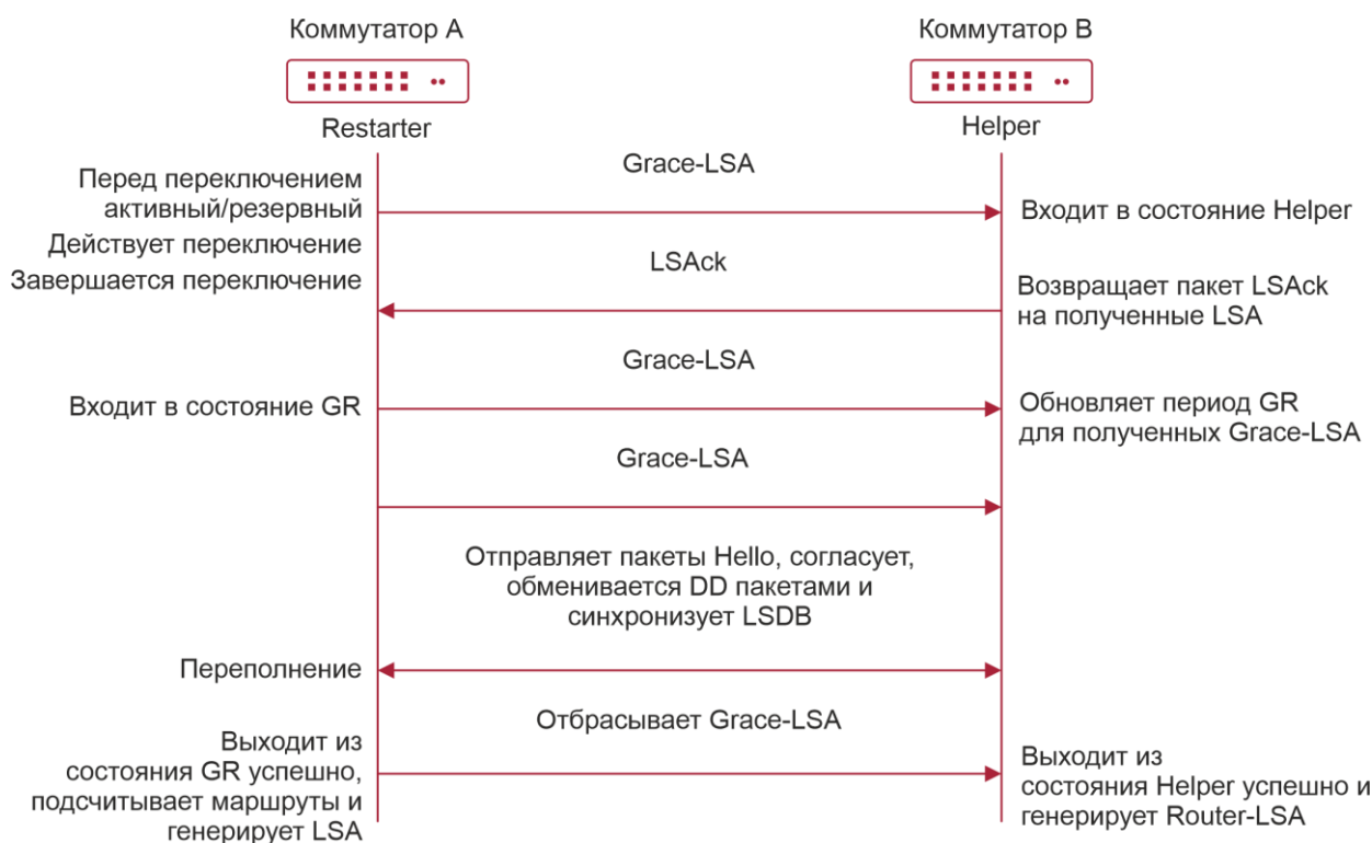
Рисунок 5-7. Обычный процесс GR OSPF
