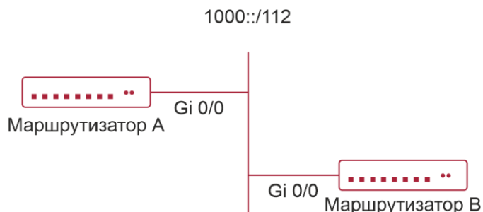
Рисунок 6-11. Топология broadcast-канала IS-ISv6
