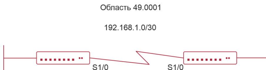
Рисунок 6-9. Топология канала P2P
