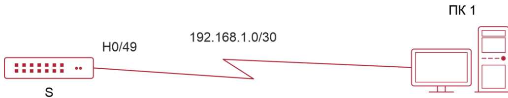
Рисунок 9-8. Топология One-to-one
