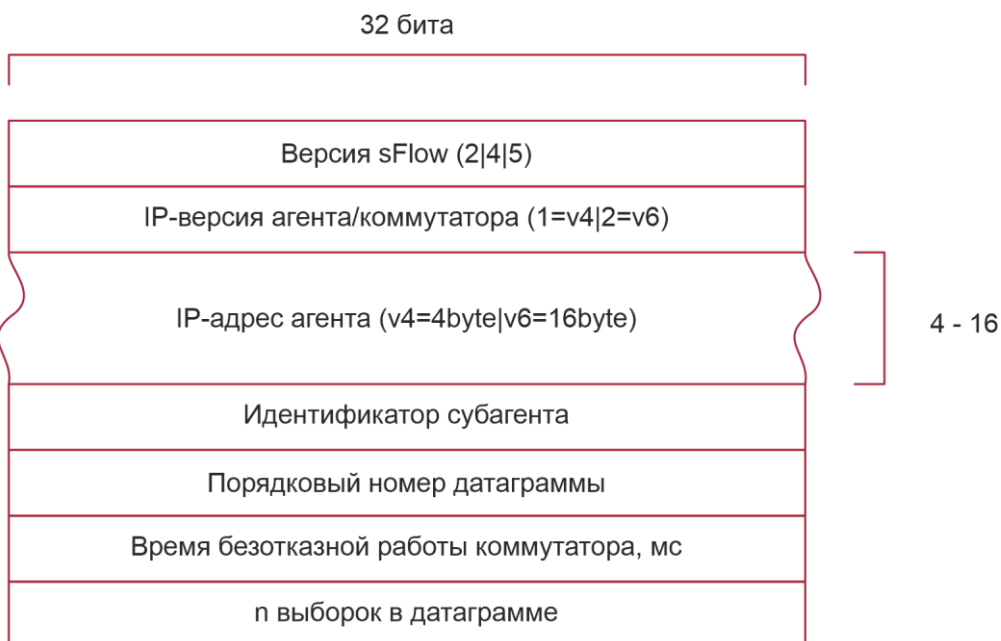
Рисунок 7-3. Заголовок sFlow
