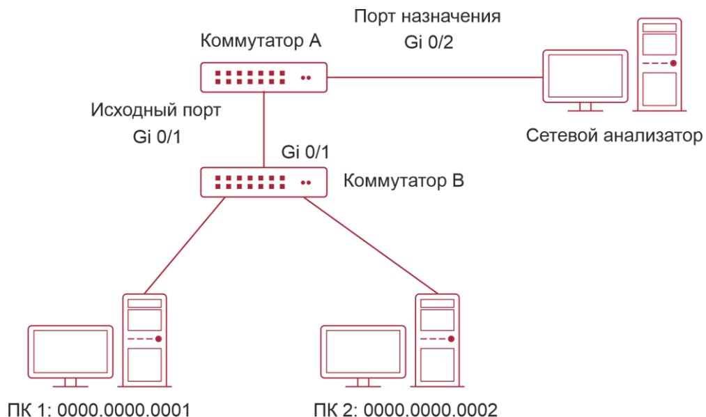
Рисунок 5-2. Топология простого приложения SPAN
