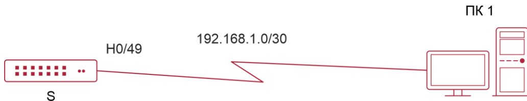
Рисунок 9-12. Топология One-to-one
