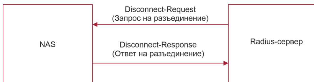
Рисунок 2-3. Обмен сообщениями DM протокола расширения динамической авторизации RADIUS
