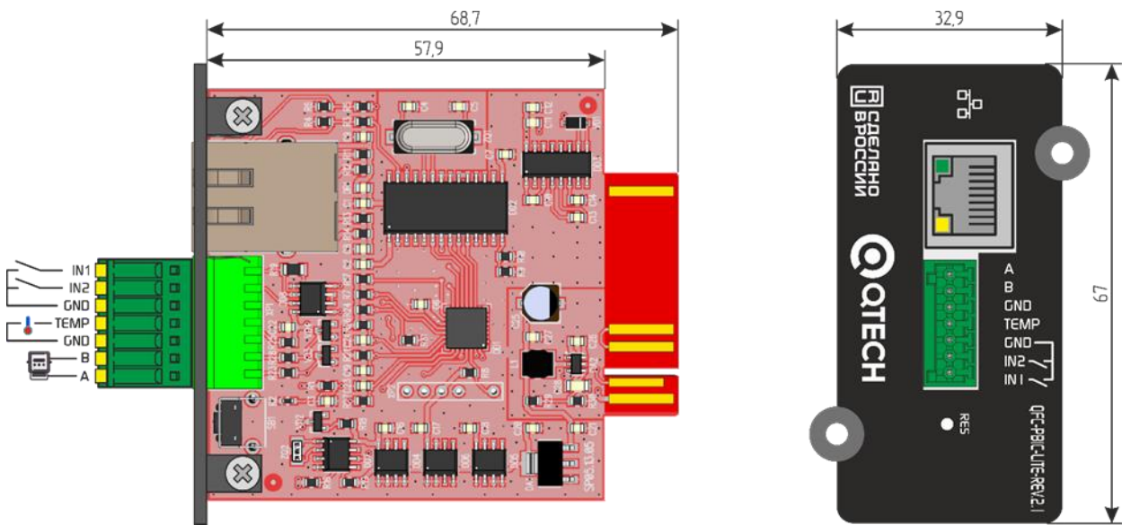
Рисунок 1-2. QFC-PBIC-LITE-REV.2.1
