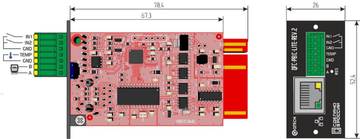
Рисунок 1-1. QFC-PBIC-LITE-REV.2
