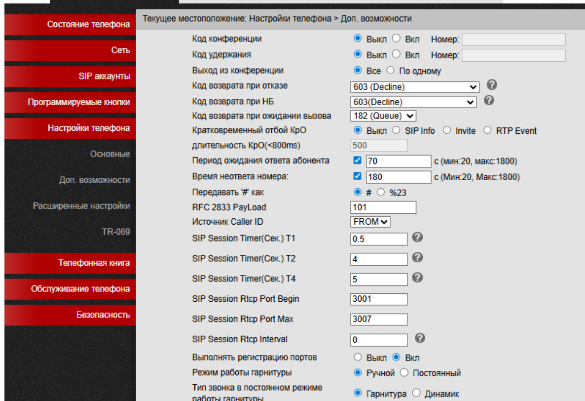
Рисунок 17 – Страница дополнительных возможностей
